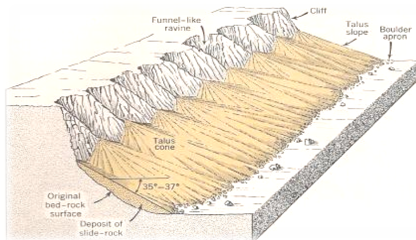
Figura 08- Material coluvial resultado de processos erosivos nas vertentes. Fonte: Strahler, 1952
