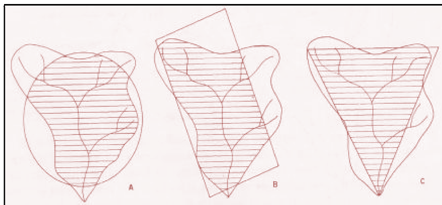
Figura 09-Geometria de bacias hidrográficas- A mensuração da forma de bacias hidrográficas conforme o procedimento estabelecido por D.R. Lee e T. Salle. No exemplo acima, o valor do índice para o círculo é de 0,313; de 0,367 para o retângulo e de 0,22 para o triângulo.
