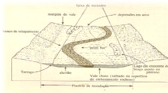
Figura 21 – Planície de Inundação ideal, com indicação dos vários componentes. Fonte: Bloom, 1996.
