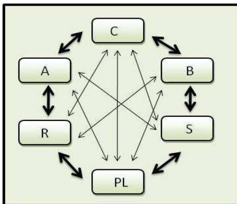
Figura 02- Esquema estrutural de um Geossistema: C = clima; A = água; R = relevo; B = biosfera; S = sociedade ; ; PL = pedosfera e litosfera.
