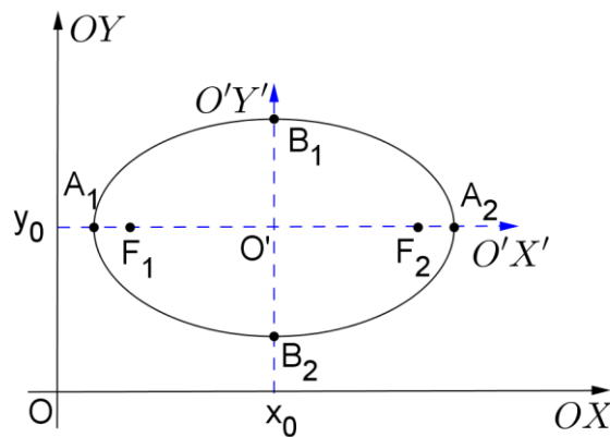
Gráfico 5 – Elipse \frac{(x-x_0)^2}{a^2} + \frac{(y-y_0)^2}{b^2} = 1
