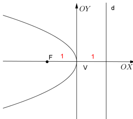
Gráfico 16 – Parábola y^2 = -4x
