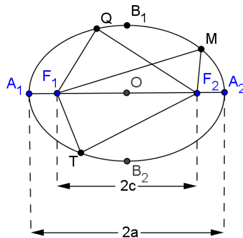
Figura 2 – Pontos da Elipse
