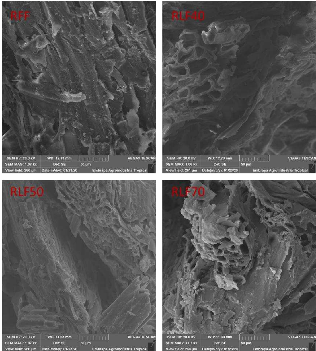
Figura 24 – Imagens de microscopia eletrônica de varredura da superfície da fratura das amostras de painéis de MDF produzidos com as resinas RFF, RLF40, RLF50 e RLF70 com uma ampliação de 1070 vezes.
