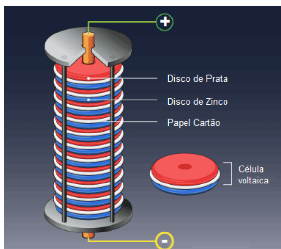
Figura 2 – Representação da pilha voltaica.
