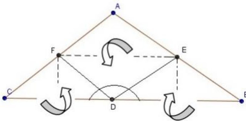
Figura 18: Construção para a demonstração da soma dos ângulos internos
