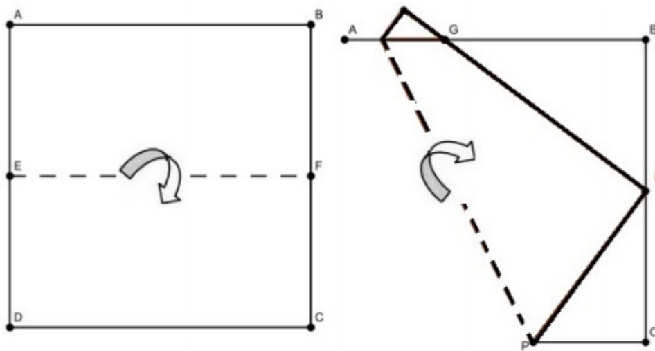
Figura 45: Construção das dobras iniciais para trisseccionar o lado do quadrado
