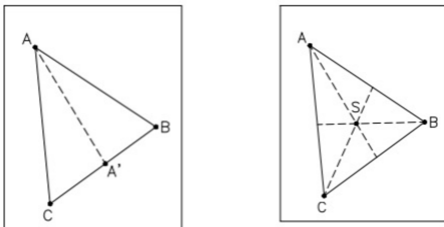
Figura 22: Construção do Incentro
