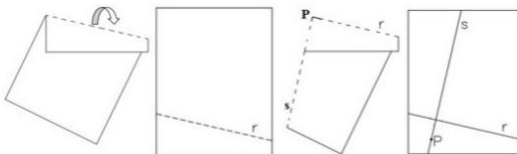
Figura 9: Retas Concorrentes
