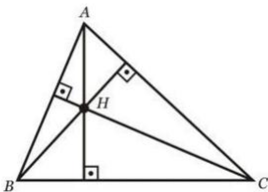
Figura 26: Construção do Ortocentro
