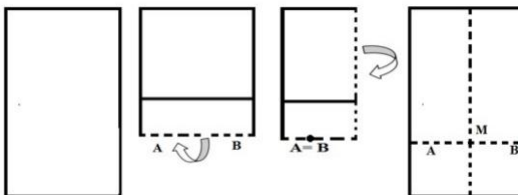
Figura 11: Ponto Médio de um Segmento
