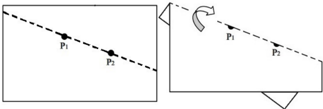
Figura 1: Construção do Axioma 1
