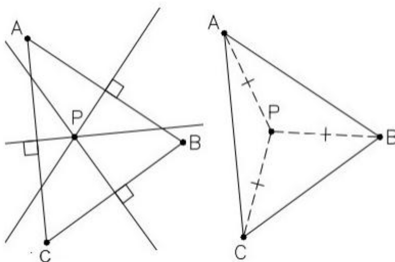
Figura 25: Circuncentro do Triângulo
