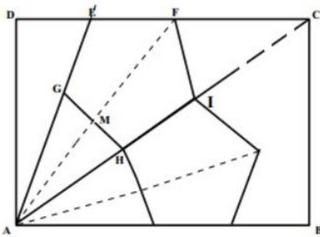
Figura 38: Pentágono Regular
