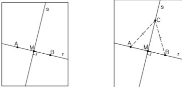
Figura 21: Construção da Reta Mediatriz
