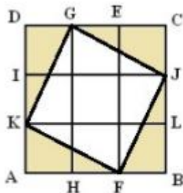
Figura 42: Teorema de Pitágoras
