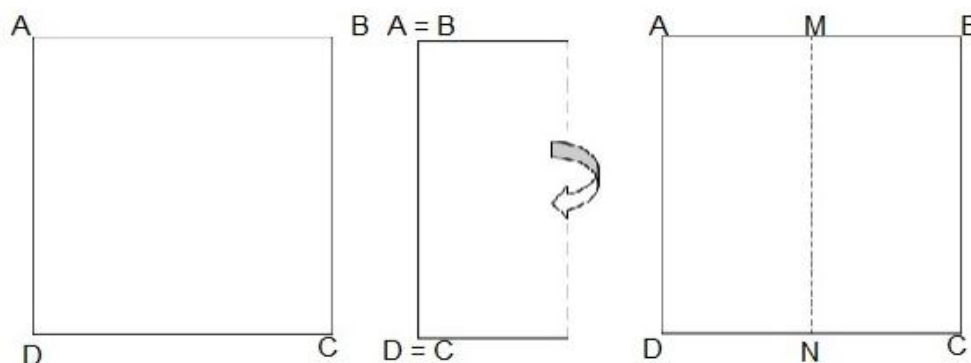
Figura 29: Construção da divisão de um segmento em 2^k partes iguais
