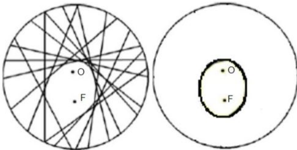
Figura 59: Construção da Elipse
