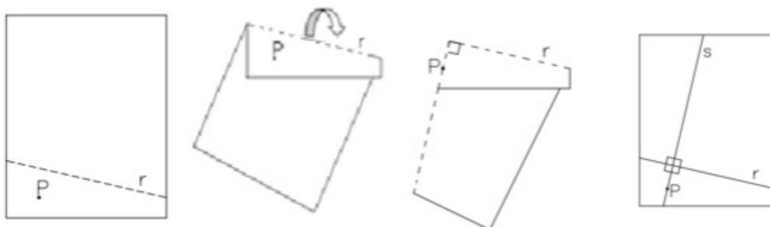
Figura 14: Retas Perpendiculares
