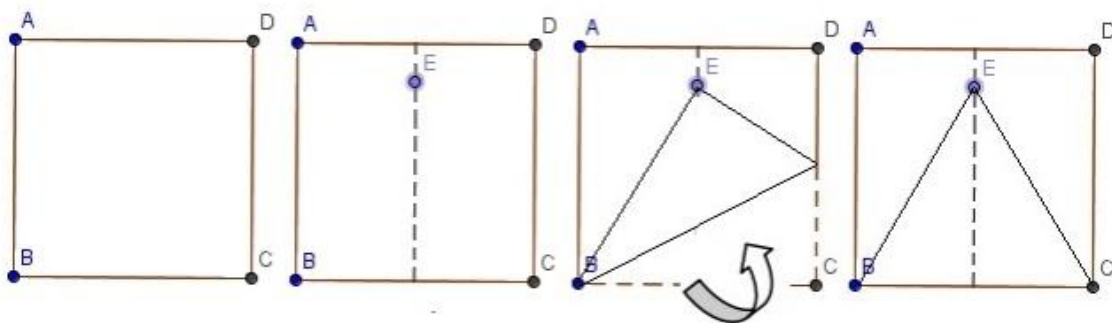
Figura 19: Construção do Triângulo Equilátero
