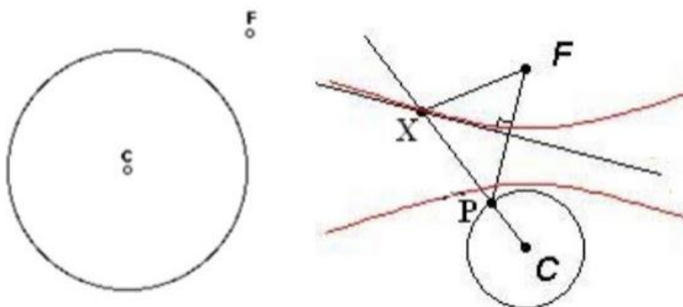
Figura 61: Construção da Hipérbole
