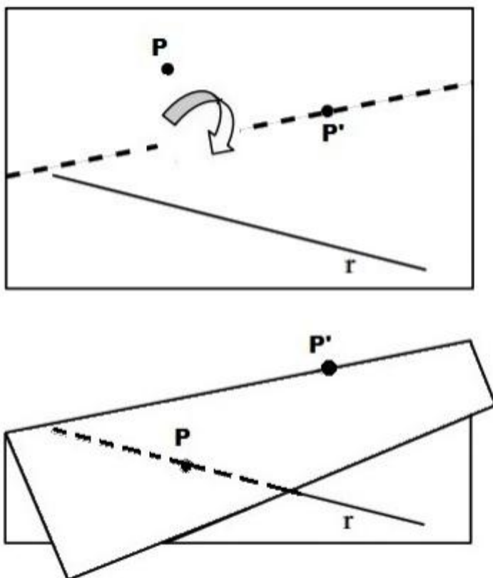
Figura 6: Construção do Axioma 5
