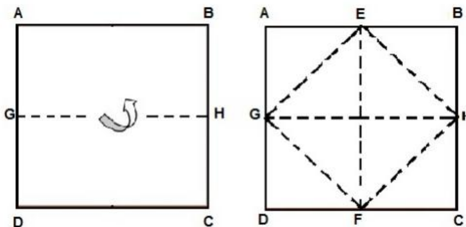
Figura 28: Um quadrado inscrito num quadrado
