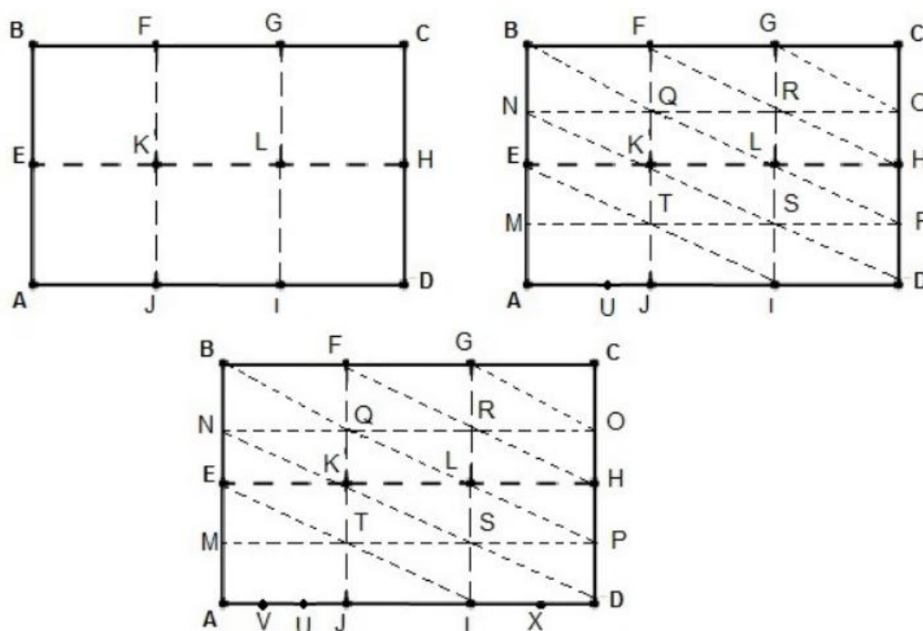
Figura 50: Retângulo com a diagonal dividindo o ângulo reto em ângulos de 54^\circ e 36^\circ
