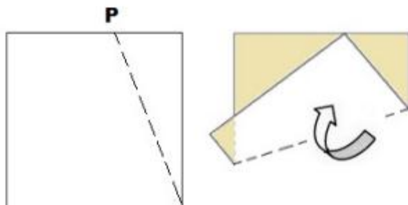
Figura 43: Dobras que formam o Teorema de Haga
