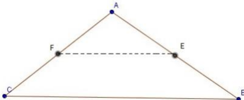
Figura 17: Construção para a demonstração da soma dos ângulos internos
