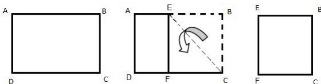
Figura 15: Quadrado construído com dobras
