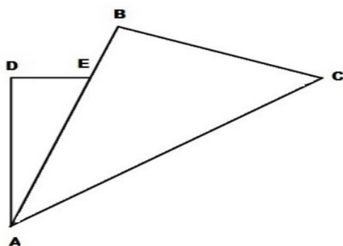
Figura 33: Dobras iniciais para a construção do pentágono regular
