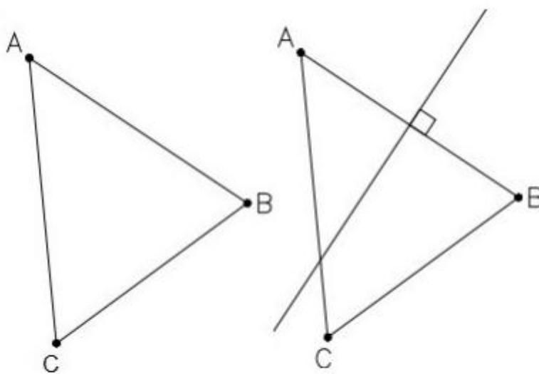
Figura 24: Circuncentro do Triângulo
