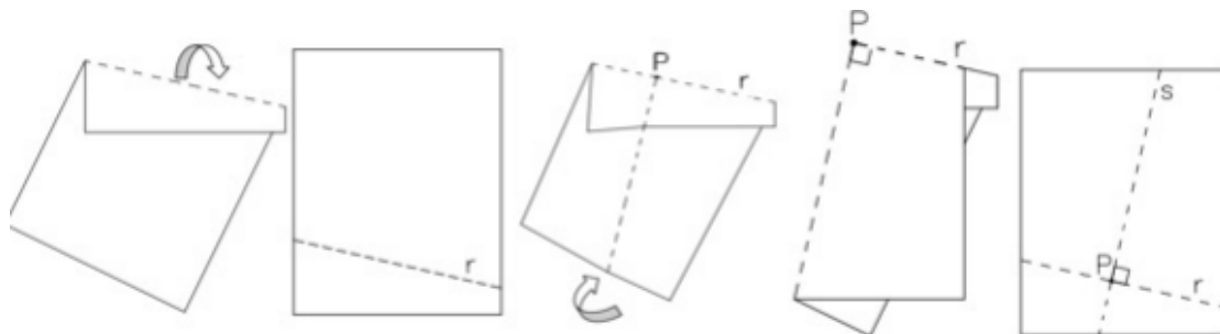
Figura 13: Dobras iniciais para a construção de Retas Perpendiculares
