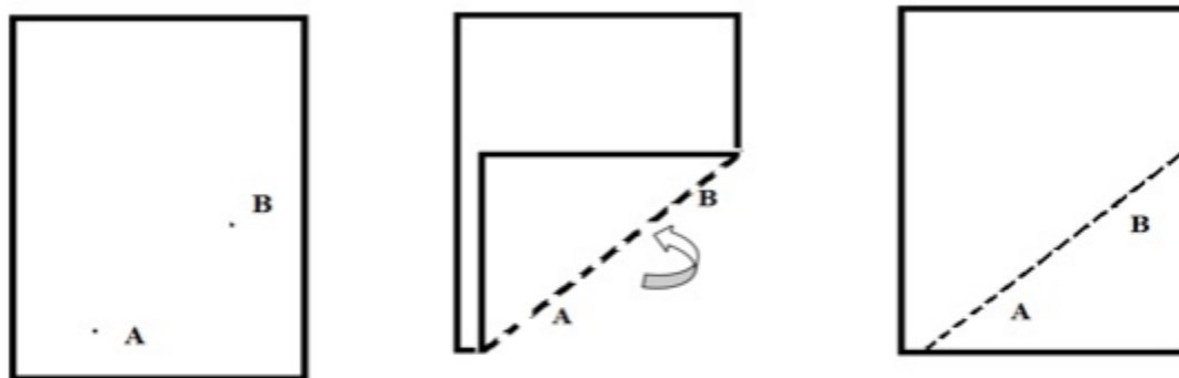
Figura 10: Reta que passa por dois pontos distintos
