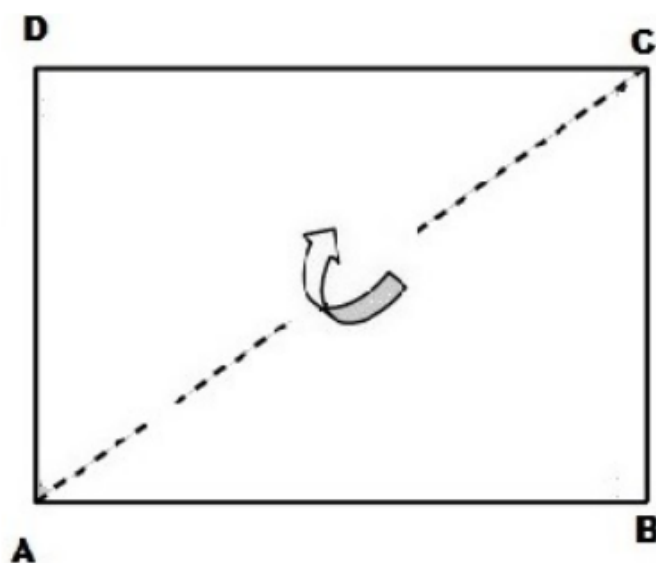
Figura 32: Dobras iniciais para a construção do pentágono regular
