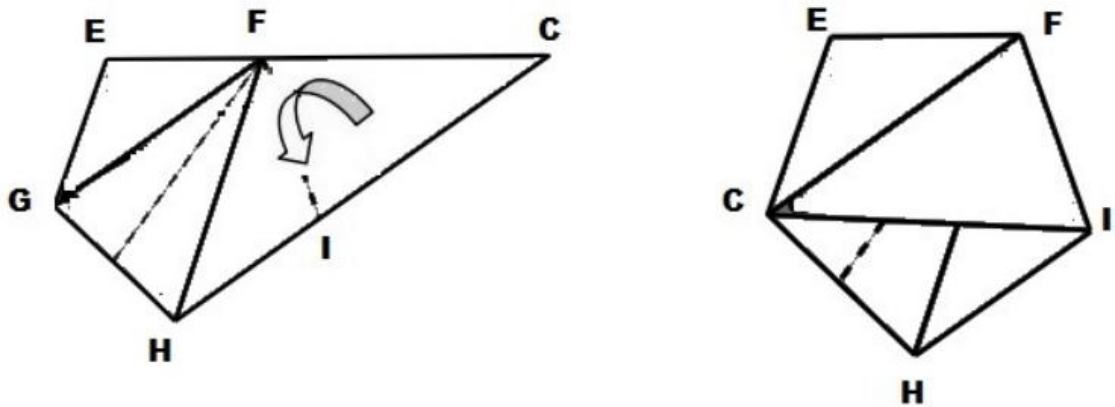
Figura 38: Pentágono Regular
