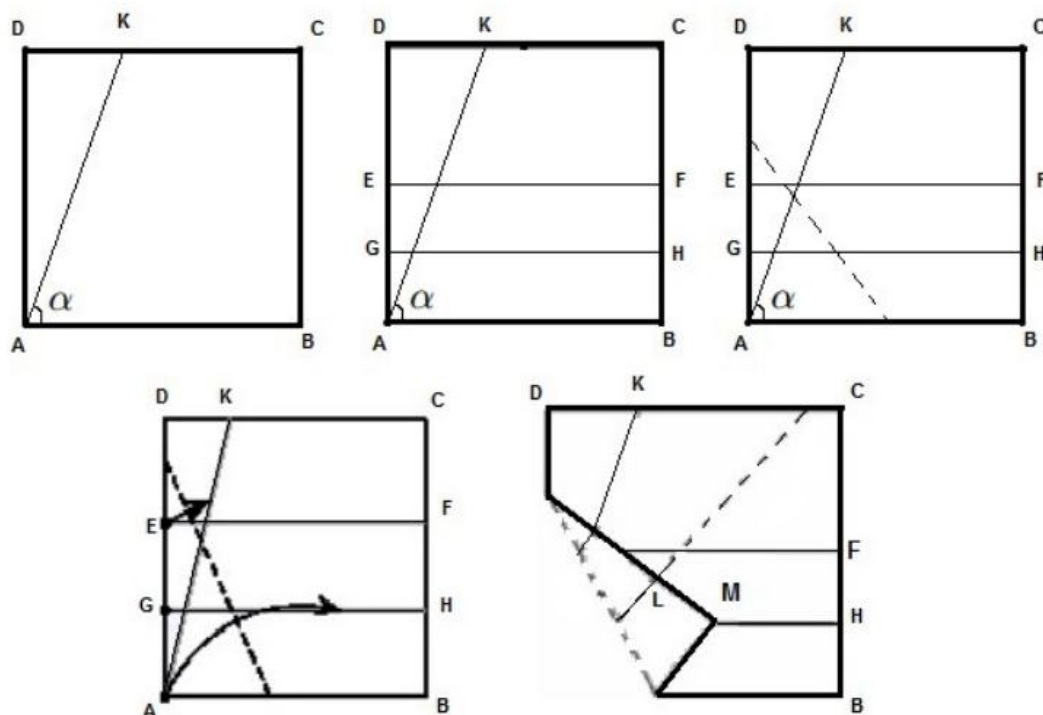
Figura 48: Dobras iniciais para a trisseção do ângulo
