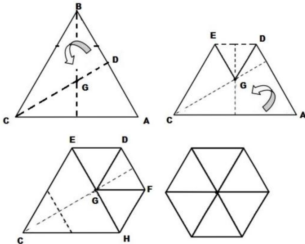
Figura 40: Construção do Hexágono regular
