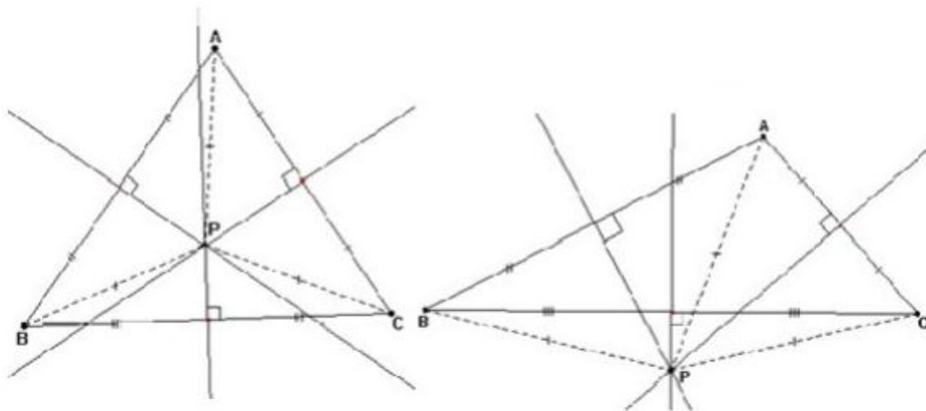
Figura 23: Construção do Circuncentro por meio de dobras
