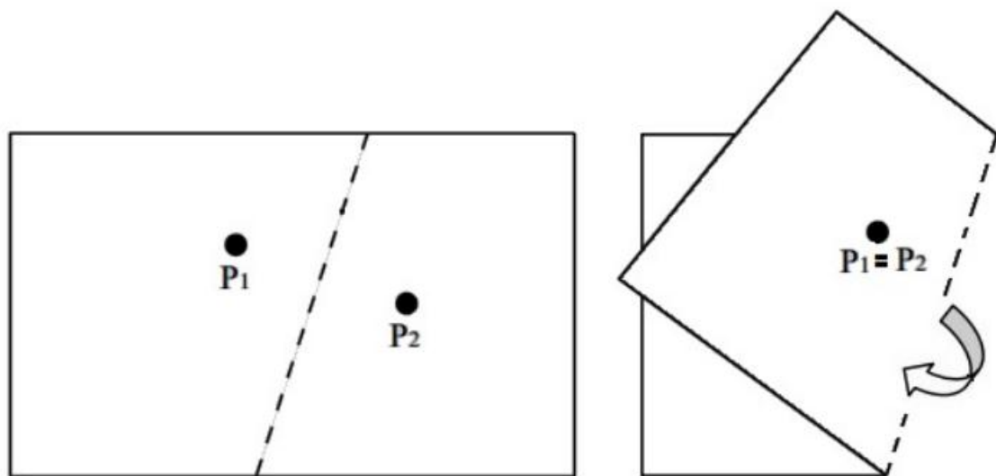
Figura 2: Construção do Axioma 2
