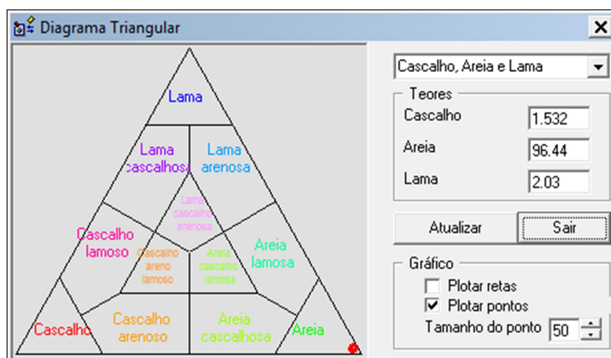
Figura 03. Resultado das análises no diagrama de Shepard (1954), realizadas com as amostras de sedimento coletadas na praia de Requenguela, Icapuí, Ceará.
