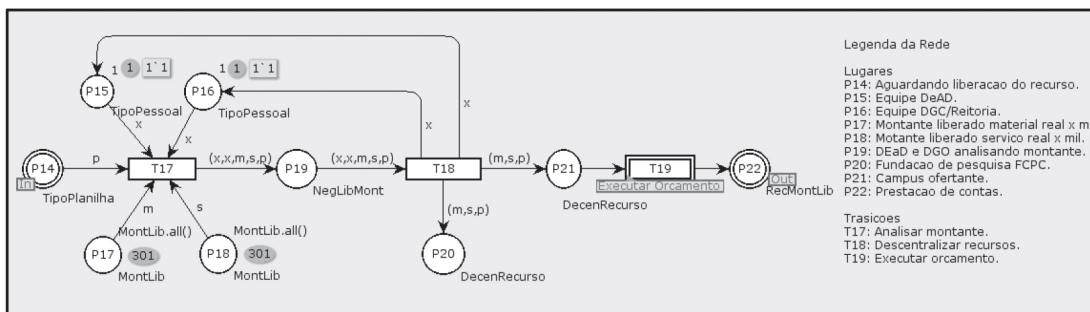
Figura 8. Sub-rede execução.
