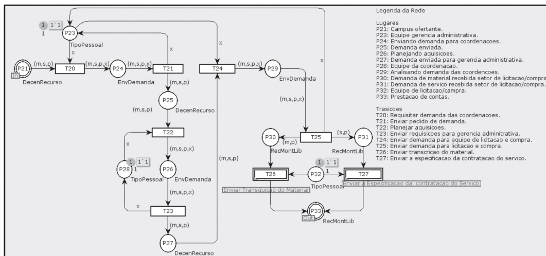
Figura 9. Executar orçamento.
