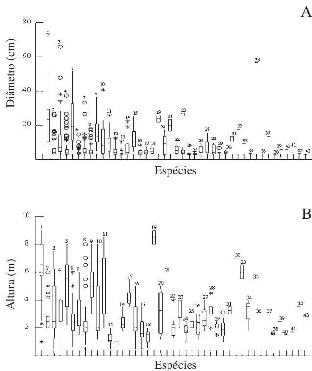
Figura 3. Espaço horizontal (A) e vertical (B) ocupado pelas espécies amostradas, ordenadas de forma decrescente pelo Valor de Cobertura (VC), no cerrado da chapada do Araripe, Barbalha, Ceará. Os números acima das barras correspondem às espécies apresentadas na Tab. 4. As linhas horizontais no interior das caixas indicam os valores da mediana. Os símbolos (*) e (O) representam valores não levados em consideração na análise (“outlines”).
