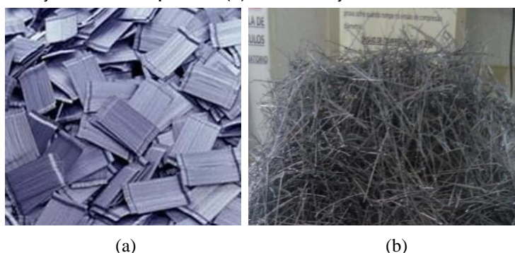
Figura 1 - (a) Fibras de aço coladas em pente e (b) fibras de aço soltas
