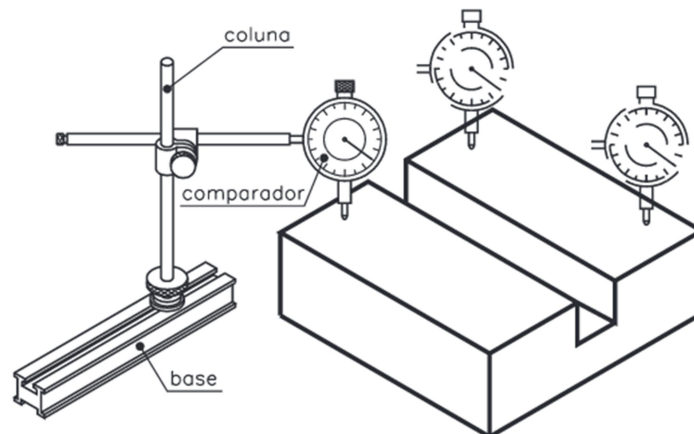
Figura 4. Posicionamento correto do relógio comparador
