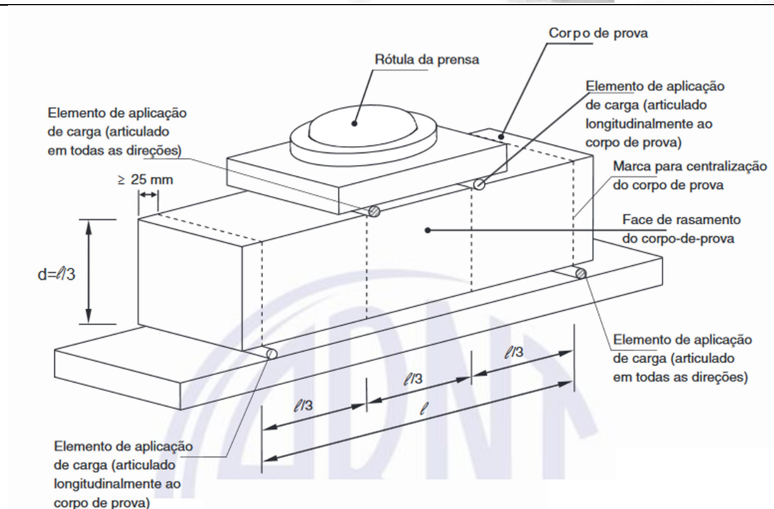
Figura 2. Dispositivo do ensaio – Perspectiva
