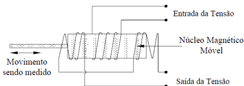
Figura 5. Esquema de LVDT
