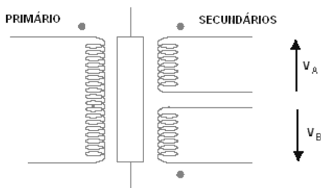
Figura 6. Esquema de um LVDT
