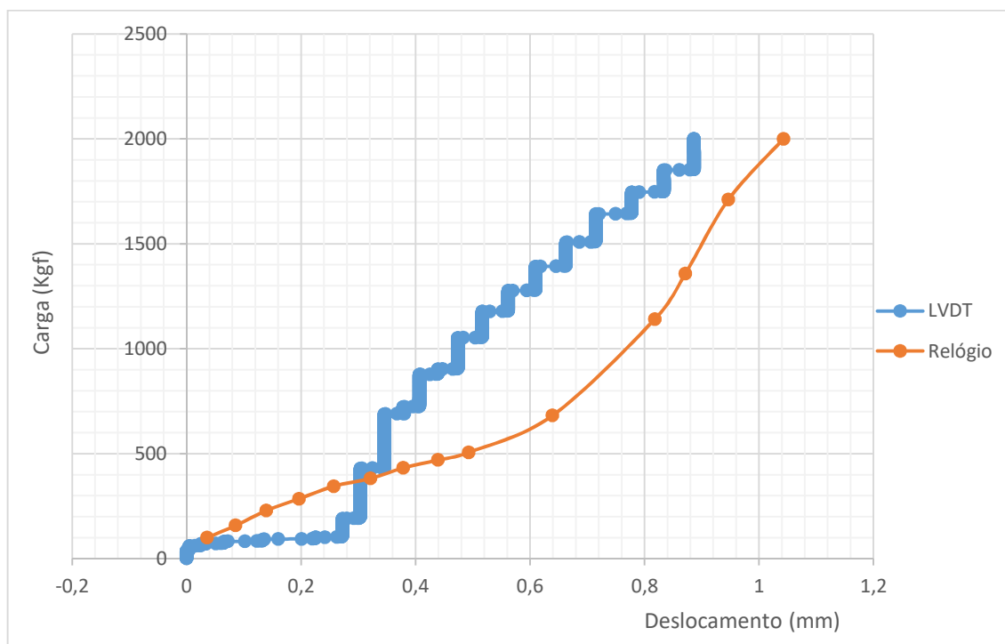
Figura 9. Comparação entre carga e deslocamento nas vigas com relógios e LVDT
