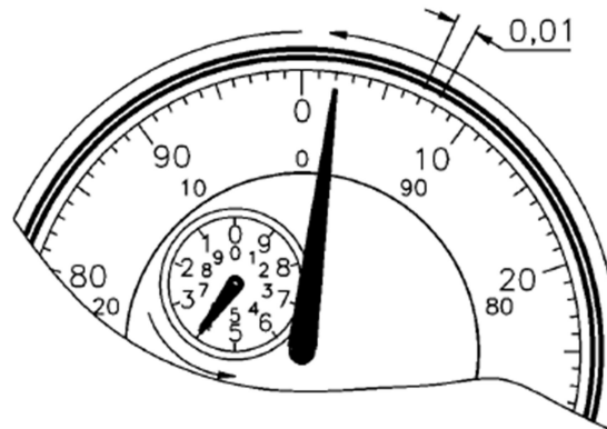
Figura 3. Leitura de um relógio
