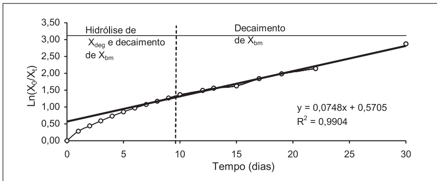
Figura 12. Linearização da curva de produção acumulada de metano durante o teste de biodegradabilidade anaeróbica do lodo. Em que: X_0 é o total degradado das frações de sólidos suspensos do lodo ( X_{deg} ) somado a X_{bm} (decaimento das bactérias) e X_t é a degradação acumulada de X_{deg} + X_{bm} em qualquer dia do ensaio.
