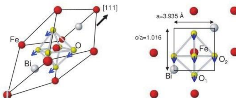
Figura 1. Esquemas de células unitárias perovskitas BiFeO_3 do tipo romboédrica e tetragonal (Wang,2003).
