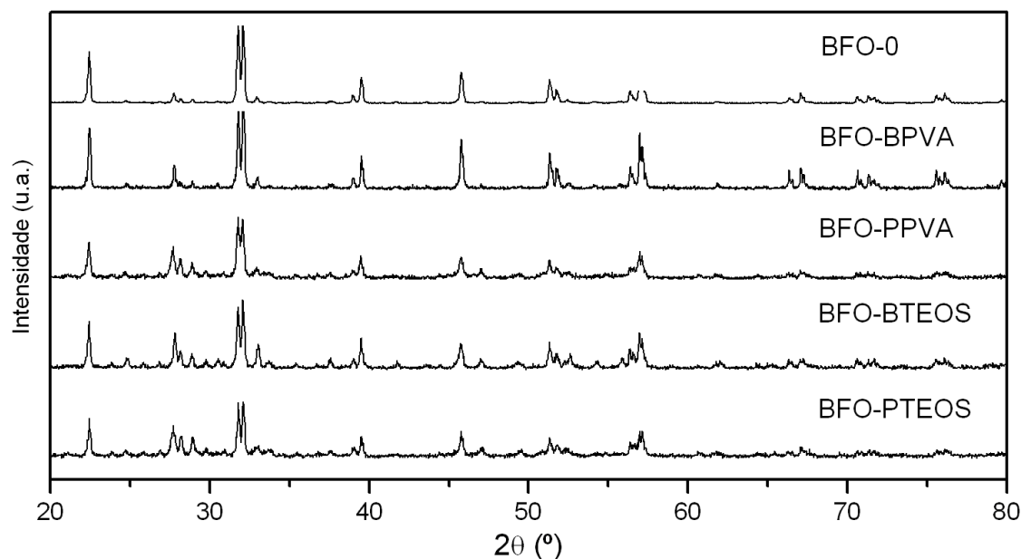
Figura 2. Padrão de difração de raios-X (DRX) das amostras sinterizadas a 810^\circ\text{C}/1\text{h} .
