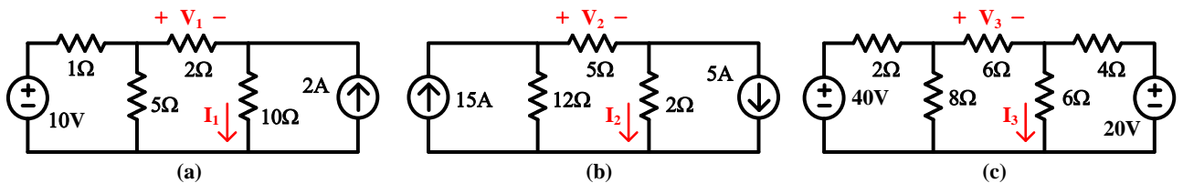
Figura 2: Circuitos propostos para análise dos métodos.
