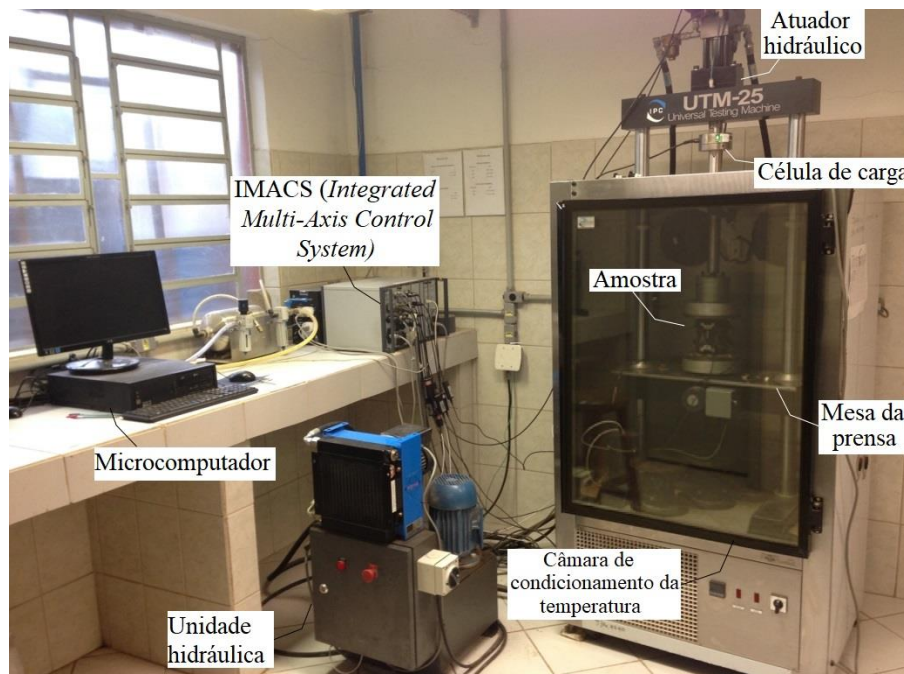
Figura 2: Prensa hidráulica, UTM-25, da Universidade Federal de Santa Maria (UFSM).
