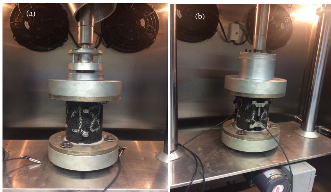
Figura 7: Sistema de ensaio de Fadiga por Tração-Compressão Direta (Uniaxial) da UFSM (a) durante montagem do aparato e (b) apto para realização do teste.
