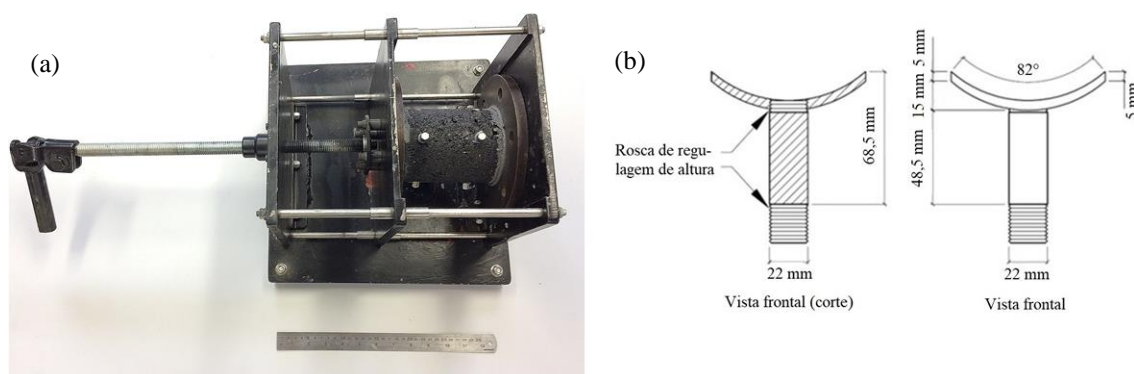
Figura 6: (a) Sistema de colagem da amostra e placas de colagem e (b) detalhamento do suporte da amostra no sistema de colagem.
