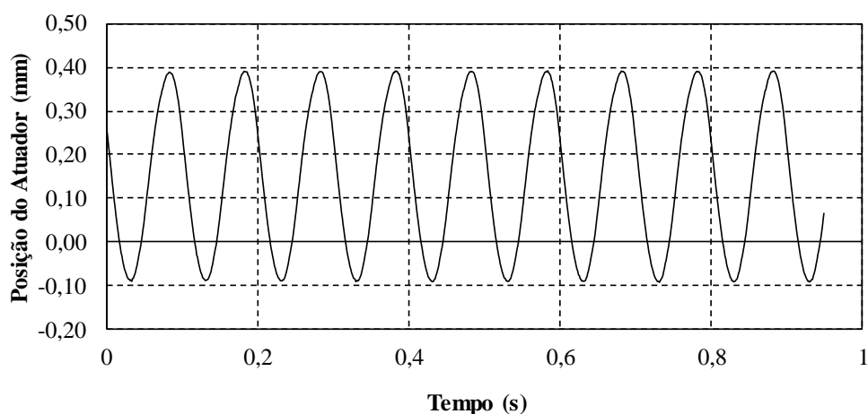
Figura 8: Leituras do LVDT do atuador durante execução do ensaio.
