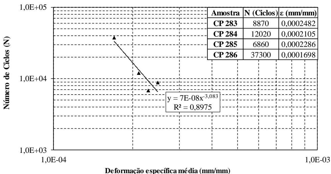
Figura 11: Relação entre desempenho de fadiga à tração e deformação específica média para diferentes ensaios de Fadiga por Tração-Compressão Direta (Uniaxial).
