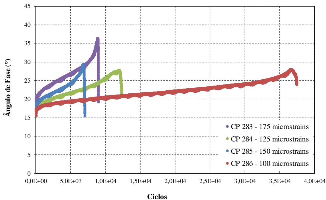
Figura 13: Relação entre o Ângulo de Fase medido ao longo dos ciclos para diferentes ensaios de Fadiga por Tração-Compressão Direta (Uniaxial).
