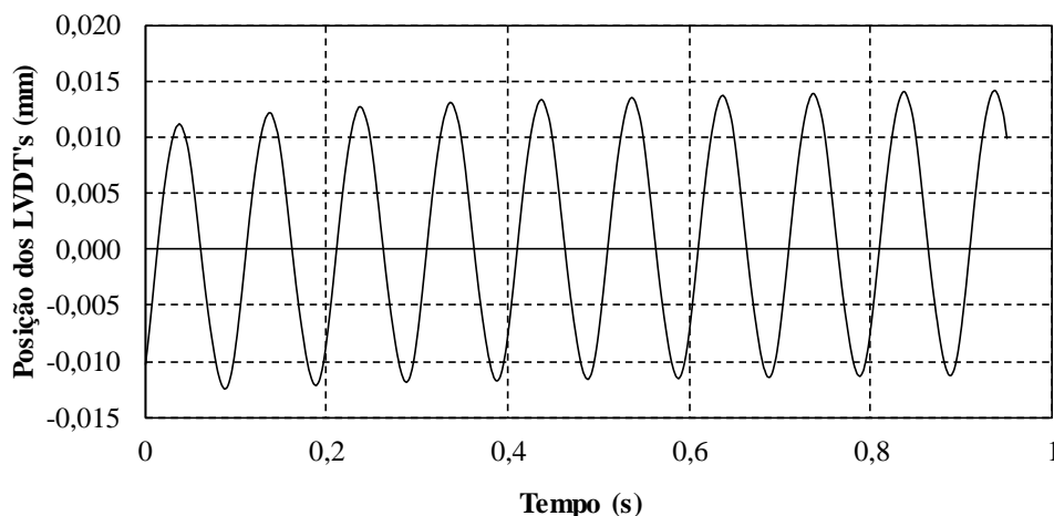
Figura 9: Leituras dos LVDTs acoplados à amostra durante execução do ensaio.
