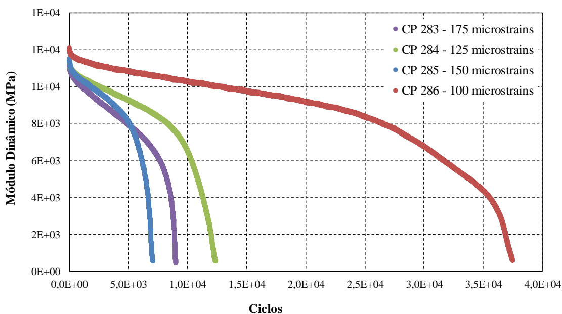
Figura 12: Relação entre o Módulo Dinâmico medido ao longo dos ciclos para diferentes ensaios de Fadiga por Tração-Compressão Direta (Uniaxial).
