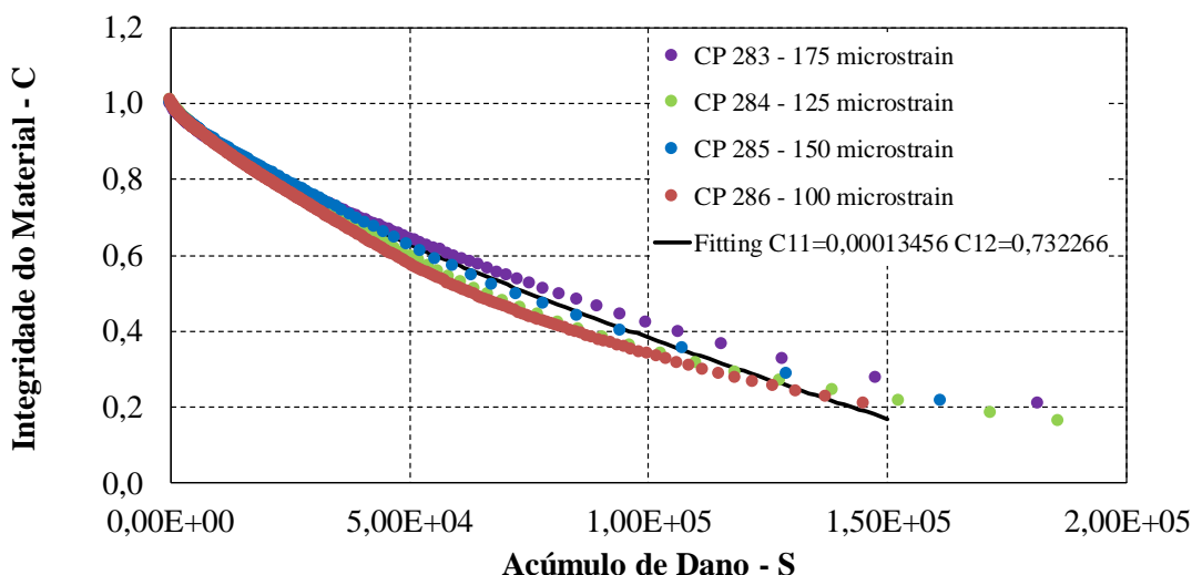
Figura 14: Curva Característica de Dano para diferentes amplitudes de deformação.
