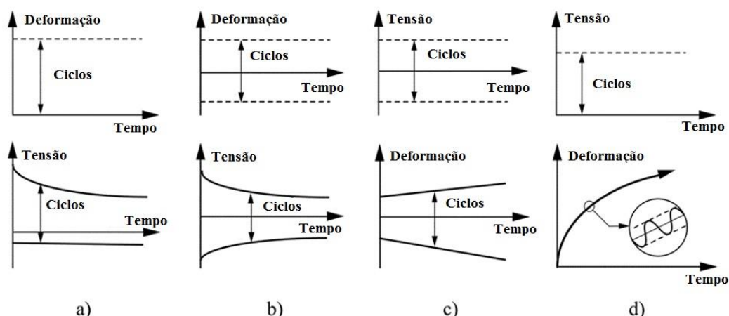
Figura 1: Esquema de representação de carregamento, deformação (a e b) ou tensão (c e d), e respectiva resposta, em tensão ou deformação [12].
