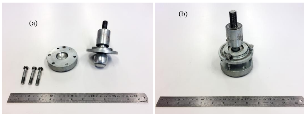
Figura 3: Sistema de rotulagem (a) desmontado e (b) montado.
