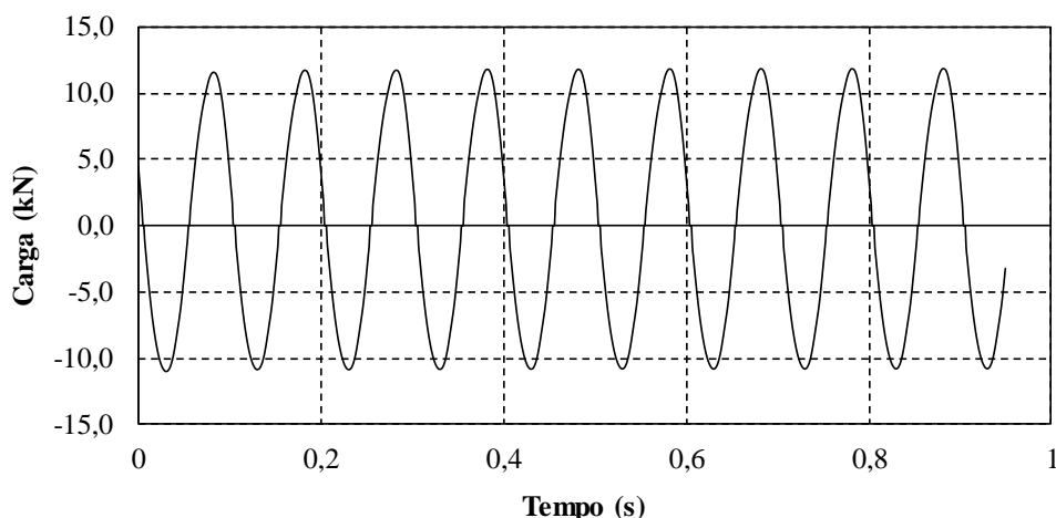
Figura 10: Leituras dos carregamentos durante execução do ensaio.
