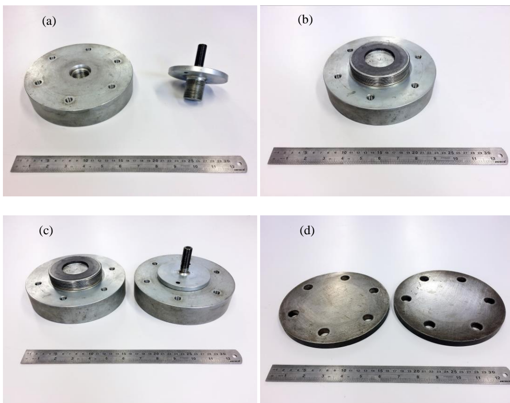
Figura 4: (a) Placa suporte inferior, (b) placa suporte superior, (c) placas de suporte e (d) placas de colagem.
