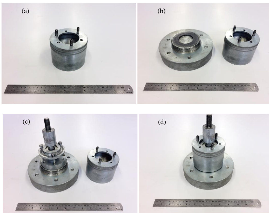
Figura 5: Copo para acoplamento do sistema de rotulagem em sequência de montagem (a, b, c e d) das peças com a placa suporte superior.
