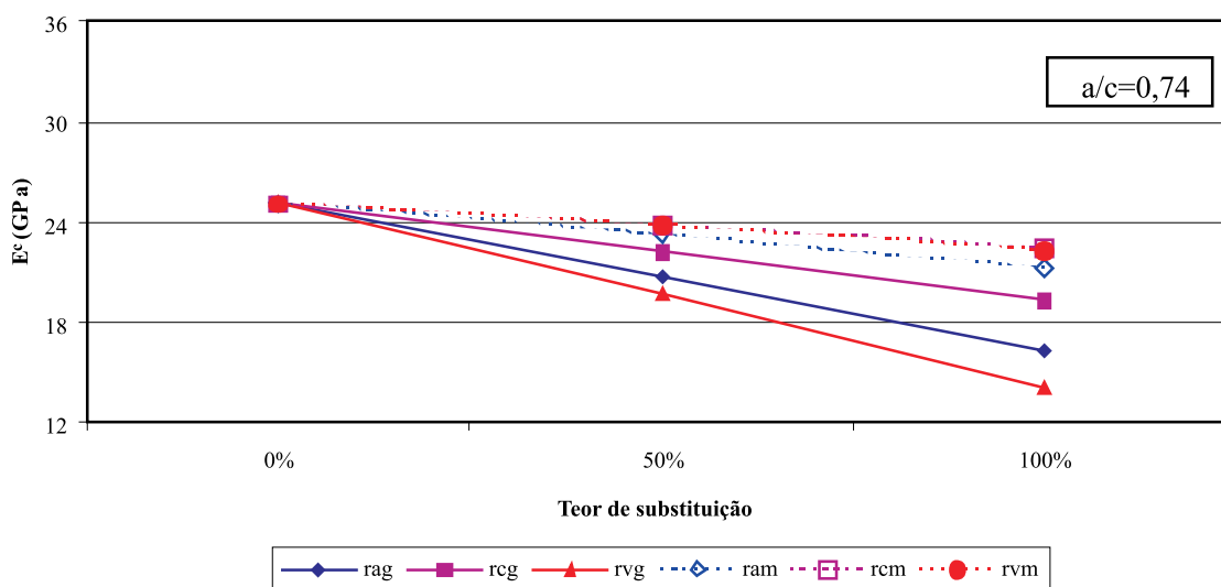
Figura 5 – Resultados de módulo de deformação em função dos teores de substituição do agregado natural pelo reciclado para a relação água/cimento igual a 0,74
