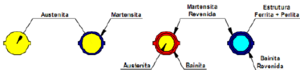
Figura 4. Esquema de fases presentes em uma barra submetida ao Thermex®
