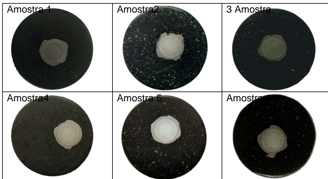
Figura 5. Macrografias Fonte: Autor.
