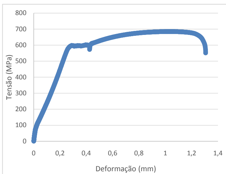
Figura 11. Tração x Deformação CR Fonte: Autor.
