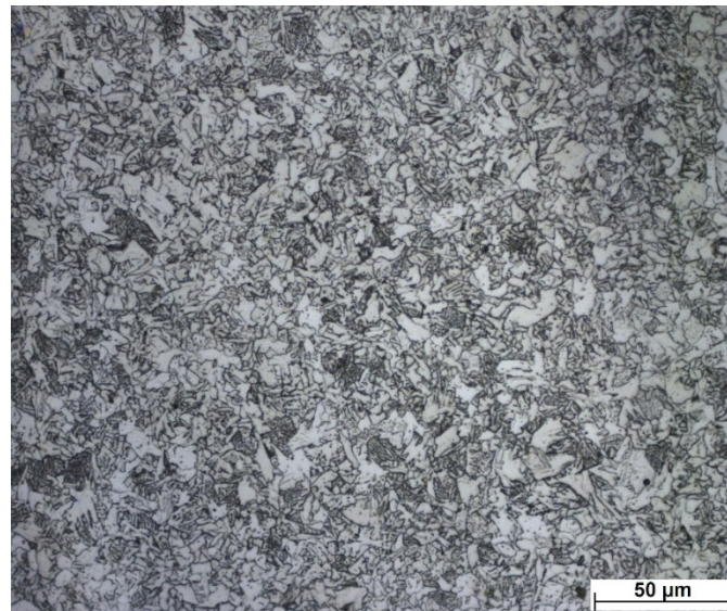
Figura 9. Micrografia camada 4 (Aumento 500x) Fonte: Autor.
