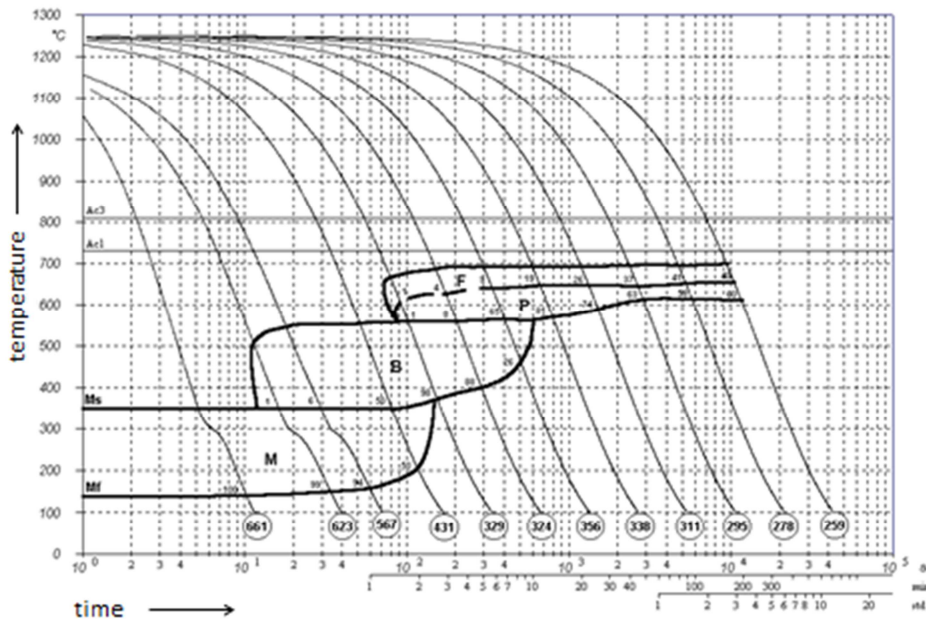
Figura 5. CCT do aço microligado ao vanádio [6].
