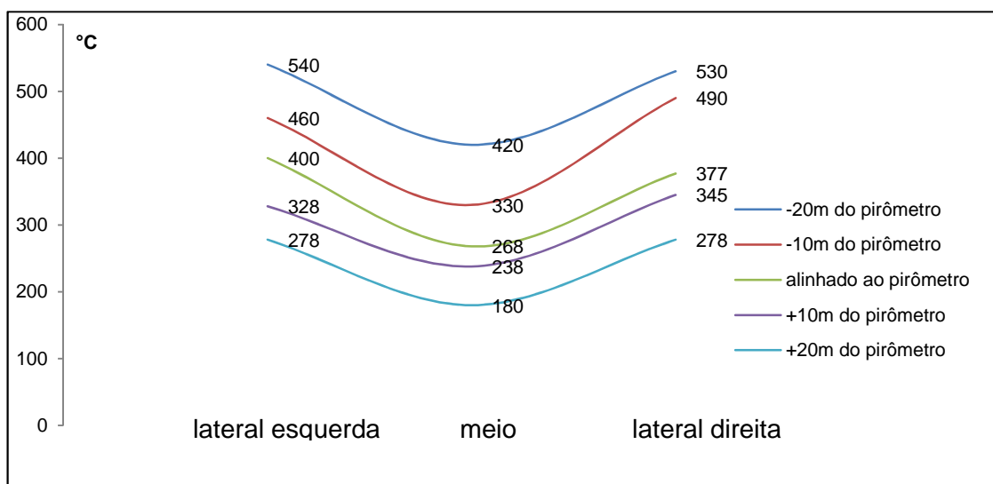
Figura 6. Variação da temperatura entre as zonas ao longo da esteira.
