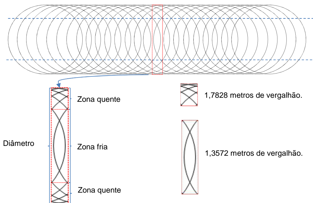
Figura 4. Esquema ilustrativo do rolo na esteira transportadora com seu elemento representativo e a divisão em zonas.
