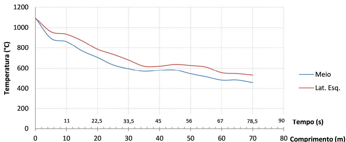
Figura 7. Curva de resfriamento ao longo da esteira com as temperaturas das zonas e tempos.
