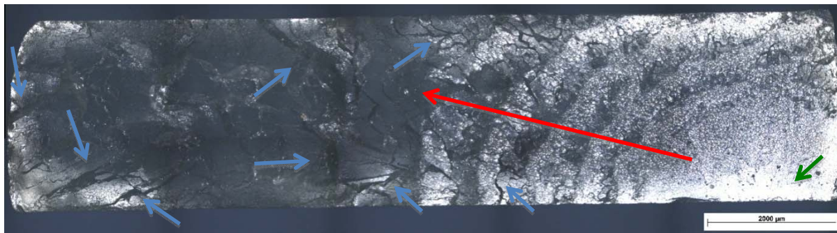
Figura 9: Superfície de fratura, grupo 2, aumento de 50x.
