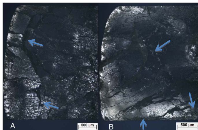
Figura 11: Detalhe no final da fratura mostrando microtrincas (seta azul), aumento de 50x: (a) grupo 1 e (b) grupo 2.
