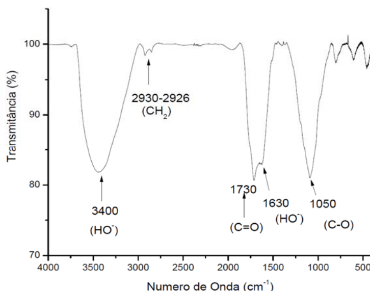
Figura 1. FTIR dos nanowhiskers obtidos.
