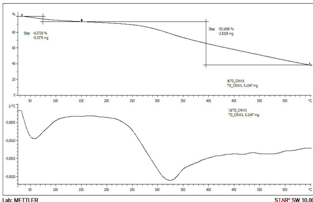
Figura 2. TG e DTG dos nanowhiskers obtidos.
