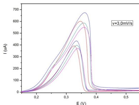
Figura 7. Análise de EPR com o AISD tratado por 10 horas.
