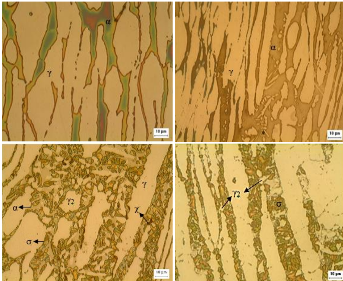
Figura 2. Microestrutura do AISD obtida por MO com magnificação de 1.000X. (a) Amostra tratada por 1 minuto. (b) Amostra tratada por 10 minutos. (c) Amostra tratada por 1 hora. (d) Amostra tratada por 10 horas.
