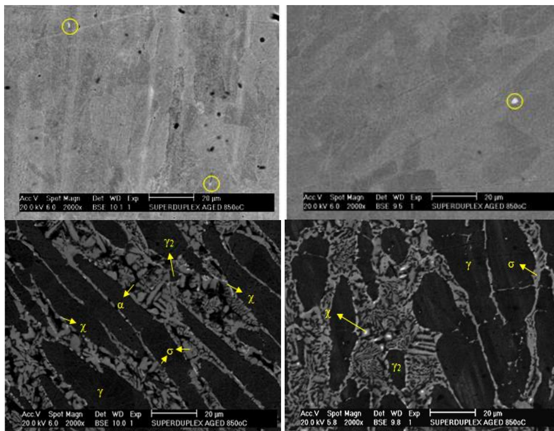
Figura 3. Micrografias das amostras de AISD tratadas termicamente. Imagens obtidas por MEV operando no modo BSE. Tempos de tratamento: (a) 1 minuto; (b) 10 minutos; (c) 1 hora; (d) 10 horas.
