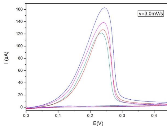
Figura 4. Ensaio de EPR-DL no AISD tratado por 1 minuto.
