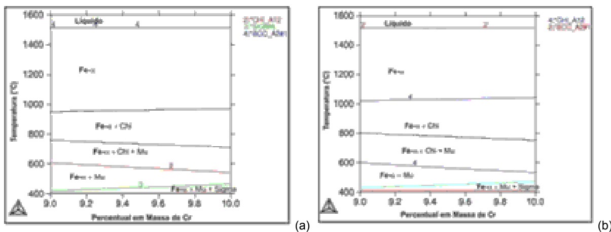
Figura 1. Diagrama de fase para as ligas. (a) Liga 1 ( 9Cr-7Mo); e (b) Liga 2 (9Cr-9Mo).
