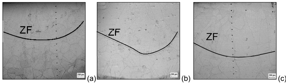
Figura 7. Micrografias da ZF da Liga 2. Aumento 50X. (a) Condição T1; (b) condição T2; e (c) condição T3.
