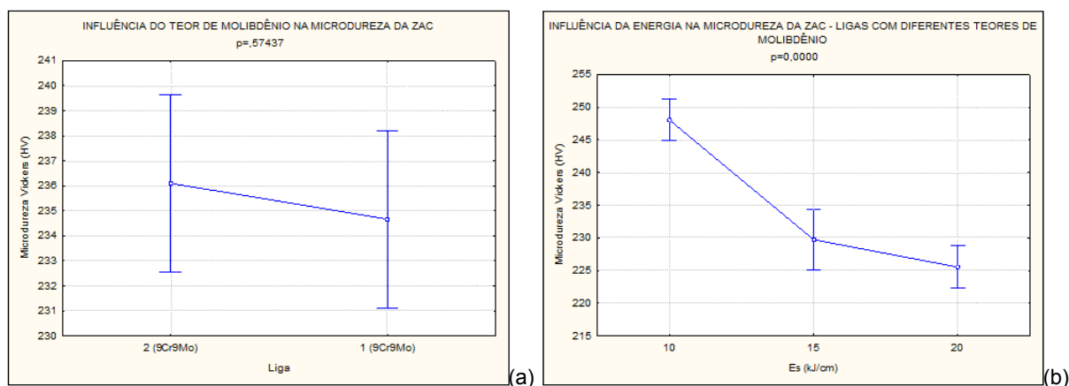
Figura 14. Análise de variância da Microdureza das ligas. (a) Influência da variação do teor de Mo; e (b) influência da energia de soldagem.
