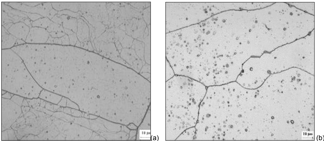
Figura 8. Micrografias das ligas após soldagem autógena. Aumento 1.000X. (a) Liga 1 condição T4; e (b) Liga 2 condição T2.
