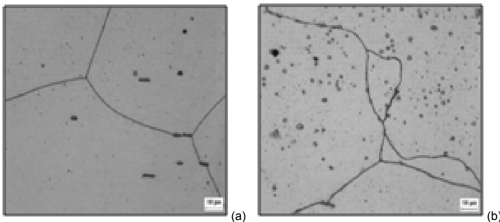
Figura 13. Micrografia dos precipitados das ligas após soldagem MIG. Aumento 1.000X. Ataque: Vilella. (a) Liga 1 - condição M4; e (b) Liga 2 - condição M3.
