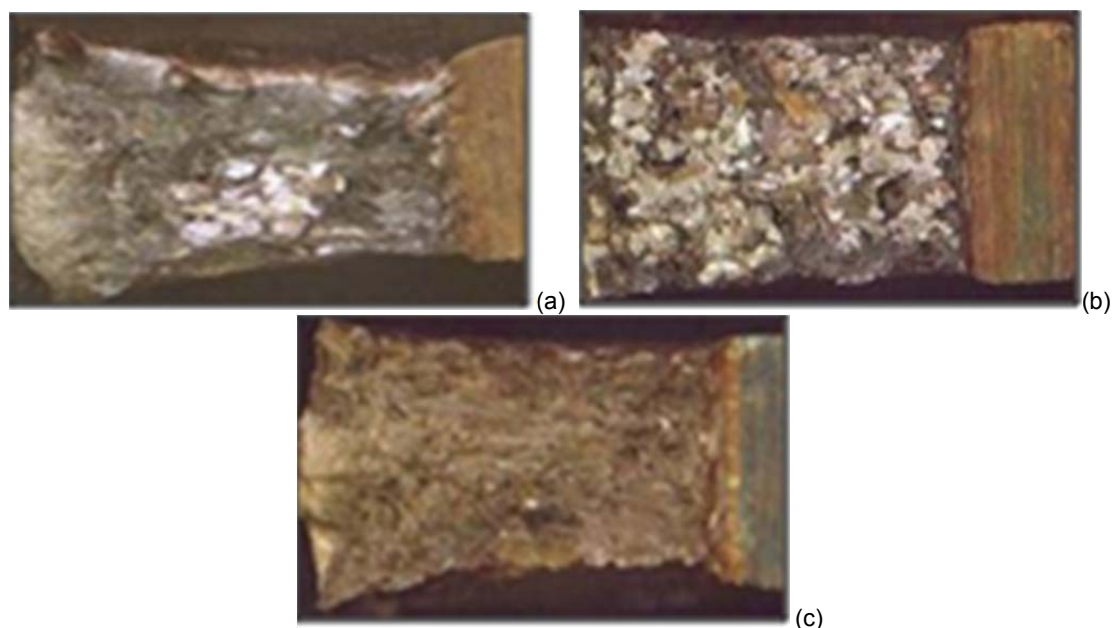
Figura 4. Aspecto da fratura dos corpos de prova Charpy-V. (a) Liga 1 (60°C); (b) Liga 2 (60°C); e (c) Liga 2 (100°C).
