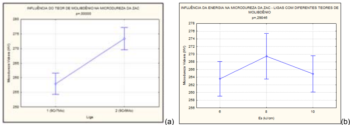
Figura 9. Análise de variância. (a) Influência do teor de Mo na microdureza da ZAC das ligas; e (b) influência da energia na microdureza da ZAC das ligas.
