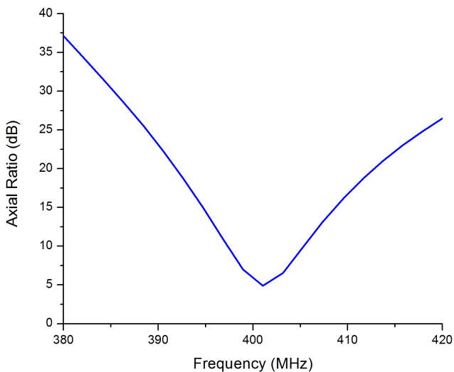
Fig. 9: Axial ratio.
