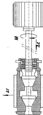
Figura 26 – Expansão por acionamento mecânico
