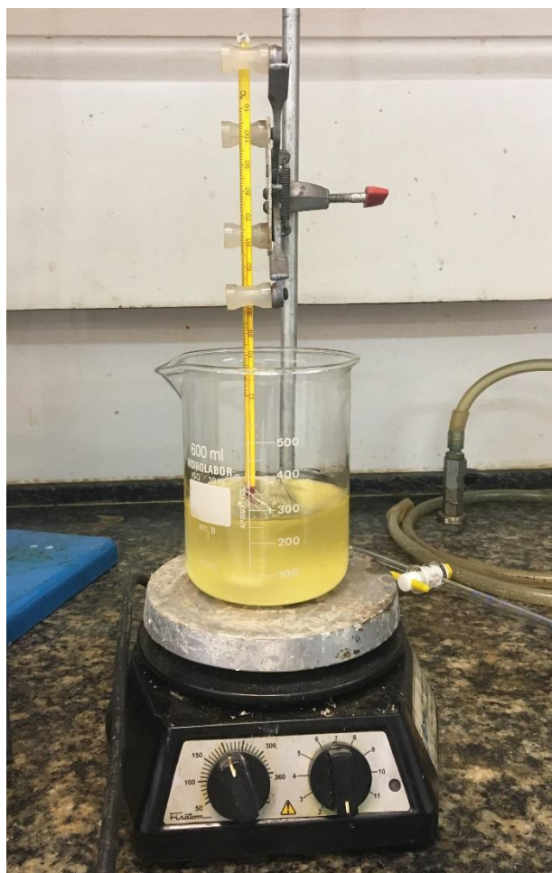
Figura 7: Processo de secagem do biodiesel de soja
