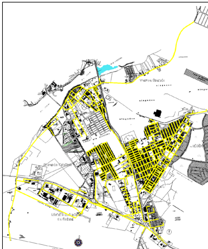
Figura 3 - Traçado da tubulação da rede no programa Autocad. Fonte: Autor, 2018.
