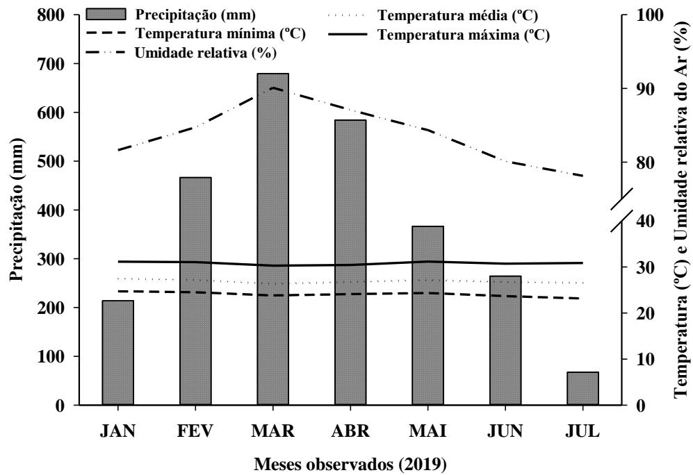
Figura 2 - Climograma do município de Fortaleza para o primeiro semestre de 2019
