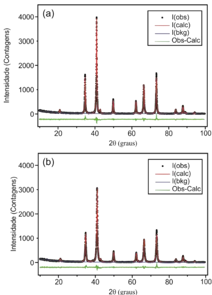
Figura 23 – Padrão de difração refinados para a amostras S4-gly com a temperatura final de calcinação em 400 °C.
