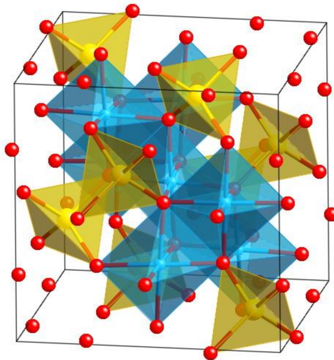
Figura 1 – Representação da organização estrutural de uma ferrita do tipo espinélio. Destacado em amarelo estão os sítios tetraédricos e em azul os sítios octaédricos. As esferas em vermelho representam os átomos de oxigênio.
