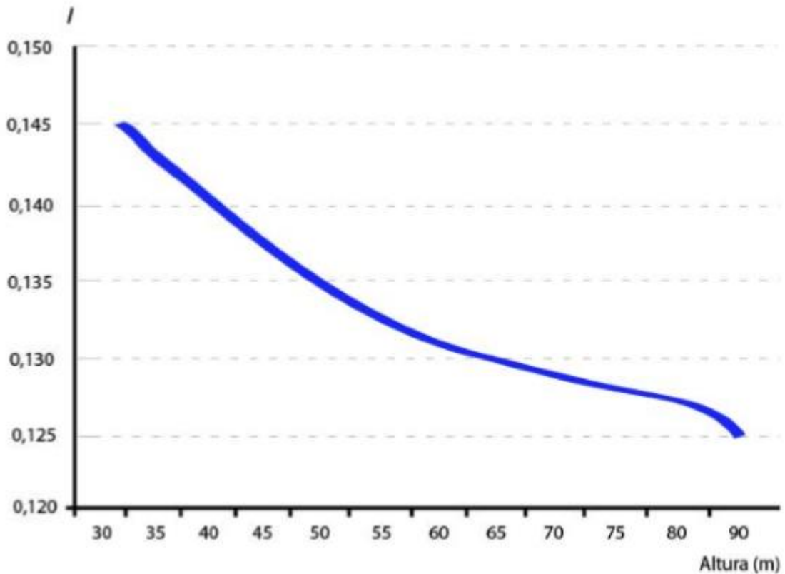
Figura 7: Variação da intensidade de turbulência pela altura.
