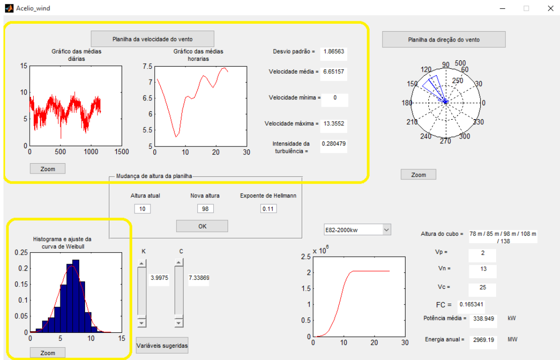
Figura 14 – Programa Acelio_wind após a entrada dos dados da velocidade dos ventos.
