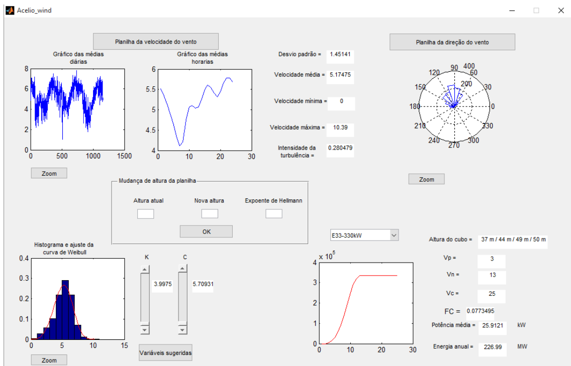
Figura 25: Simulação em uma altura de 10m para a cidade de Icapuí, para uma turbina E33-330kW.
