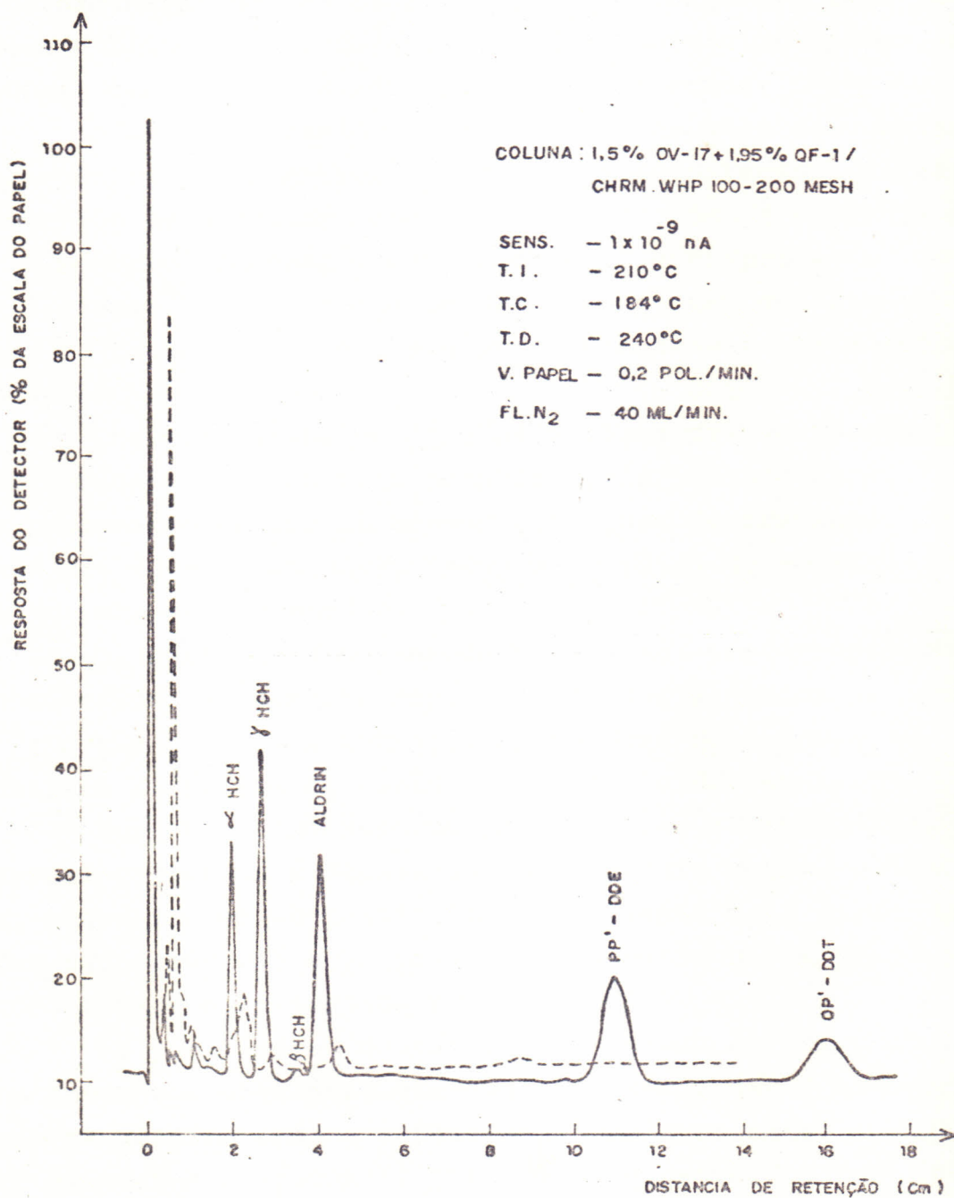
FIGURA 10 - Cromatograma obtido do branco da análise (linha pontilhada) e cromatograma de uma mistura de padrões (linha cheia)
