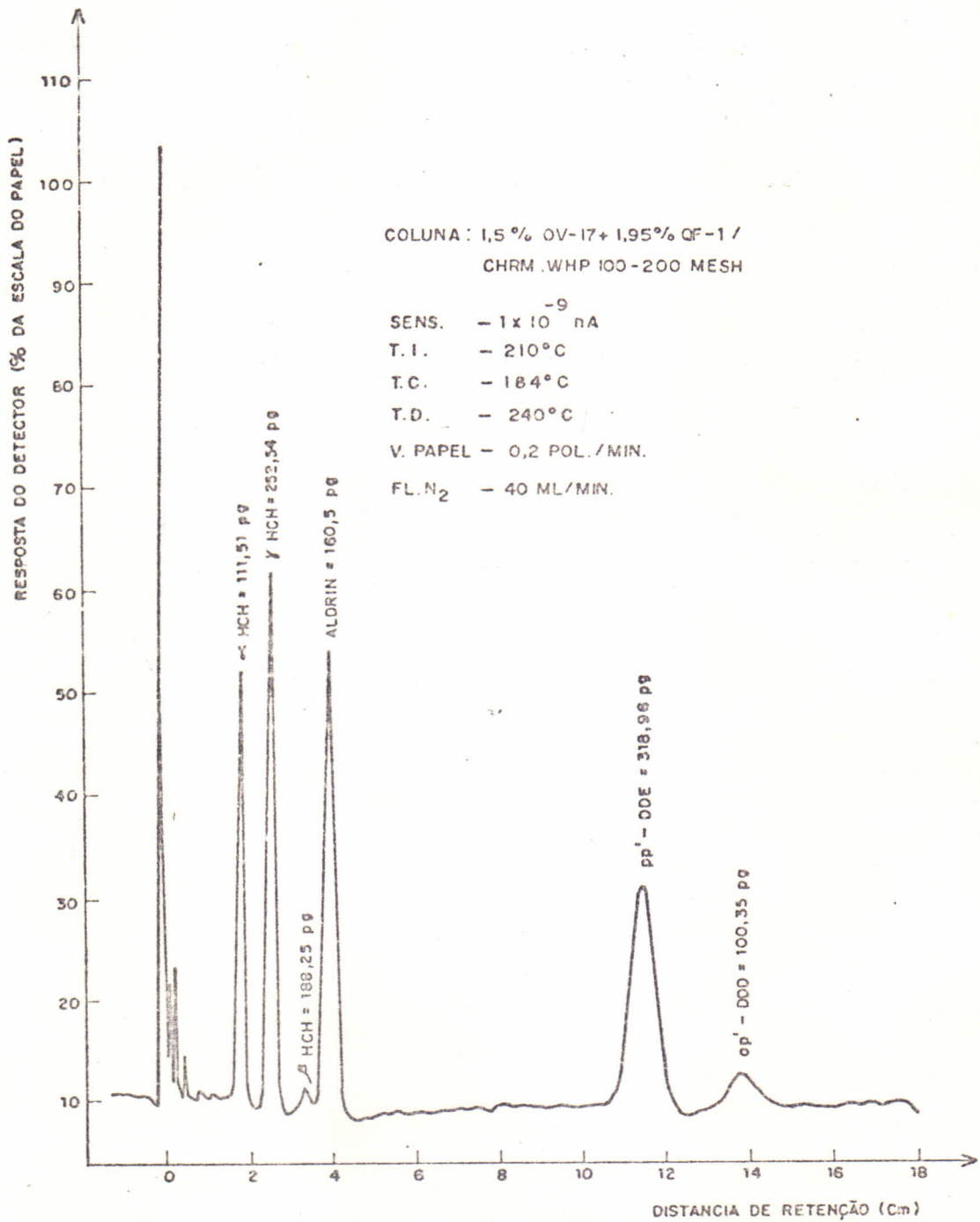
FIGURA 12 - Cromatograma obtido para uma mistura de seis padrões.
