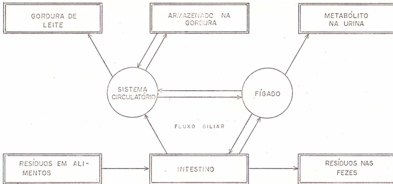
FIGURA 4 - Possíveis vias de distribuição em mamíferos dos pesticidas ingeridos como resíduos em alimentos 40 .
