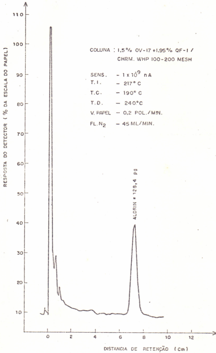
FIGURA 11 - Cromatograma obtido para o al drin.
