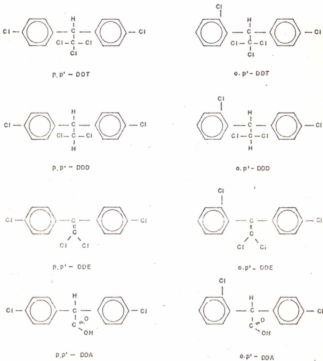
FIGURA 3 - Alguns metabólitos do DDT 4 .
