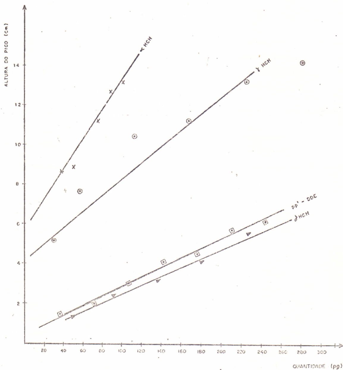
FIGURA 8 - Curva de linearidade do detector obtida para alguns pesticidas organoclorados.
