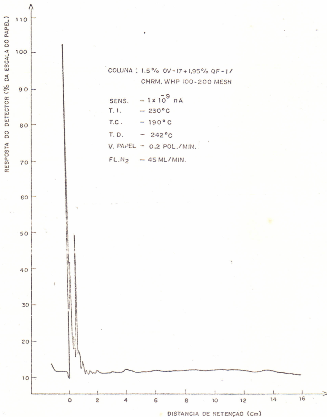
FIGURA 5 - Cromatograma obtido da alíquota de n-hexano concentrado na razão de 300:3.
