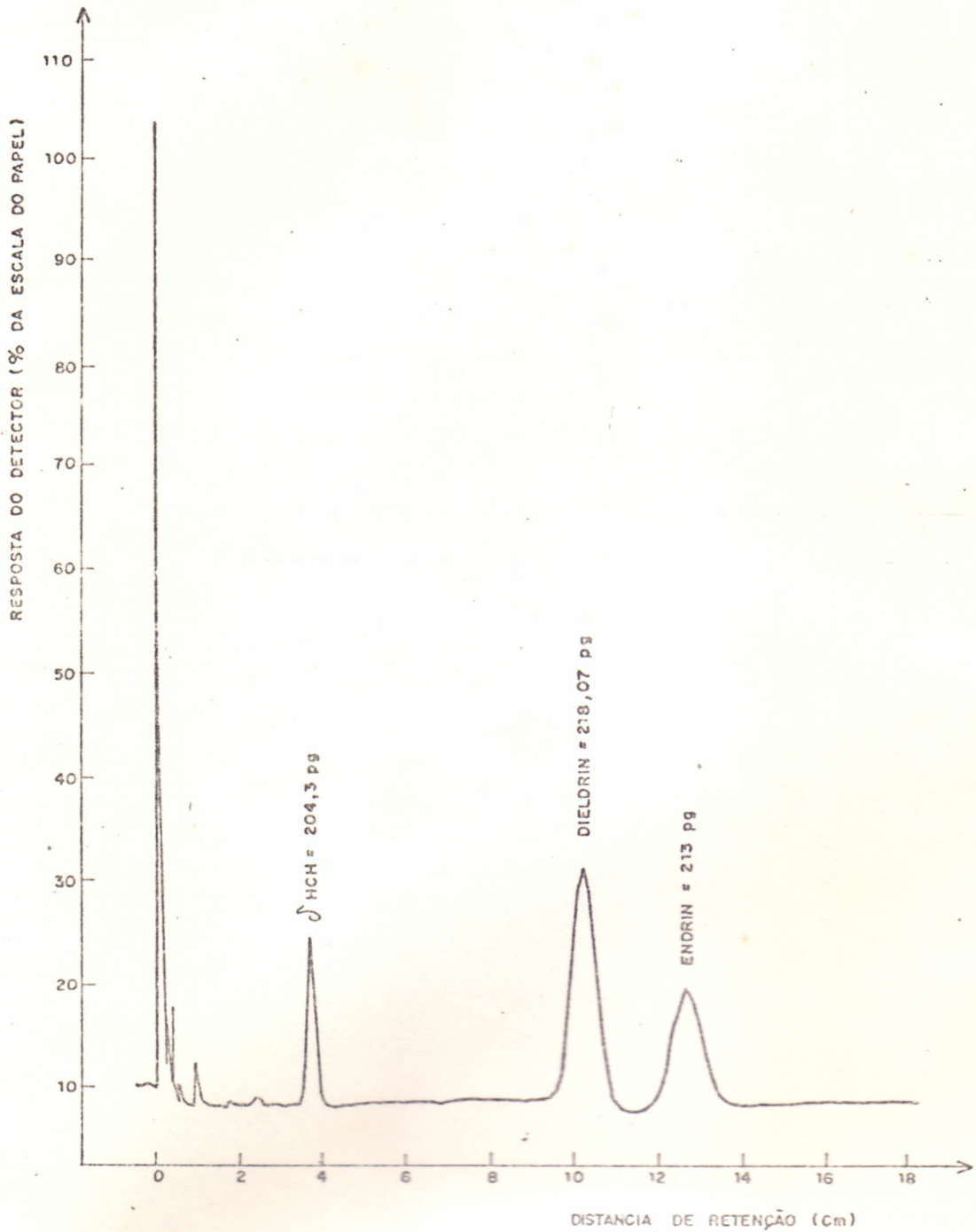
FIGURA 13 - Cromatograma obtido para uma mistura de padrões, \delta -HCH, dieldrin e endrin, nas mesmas condições descritas na FIGURA 12.
