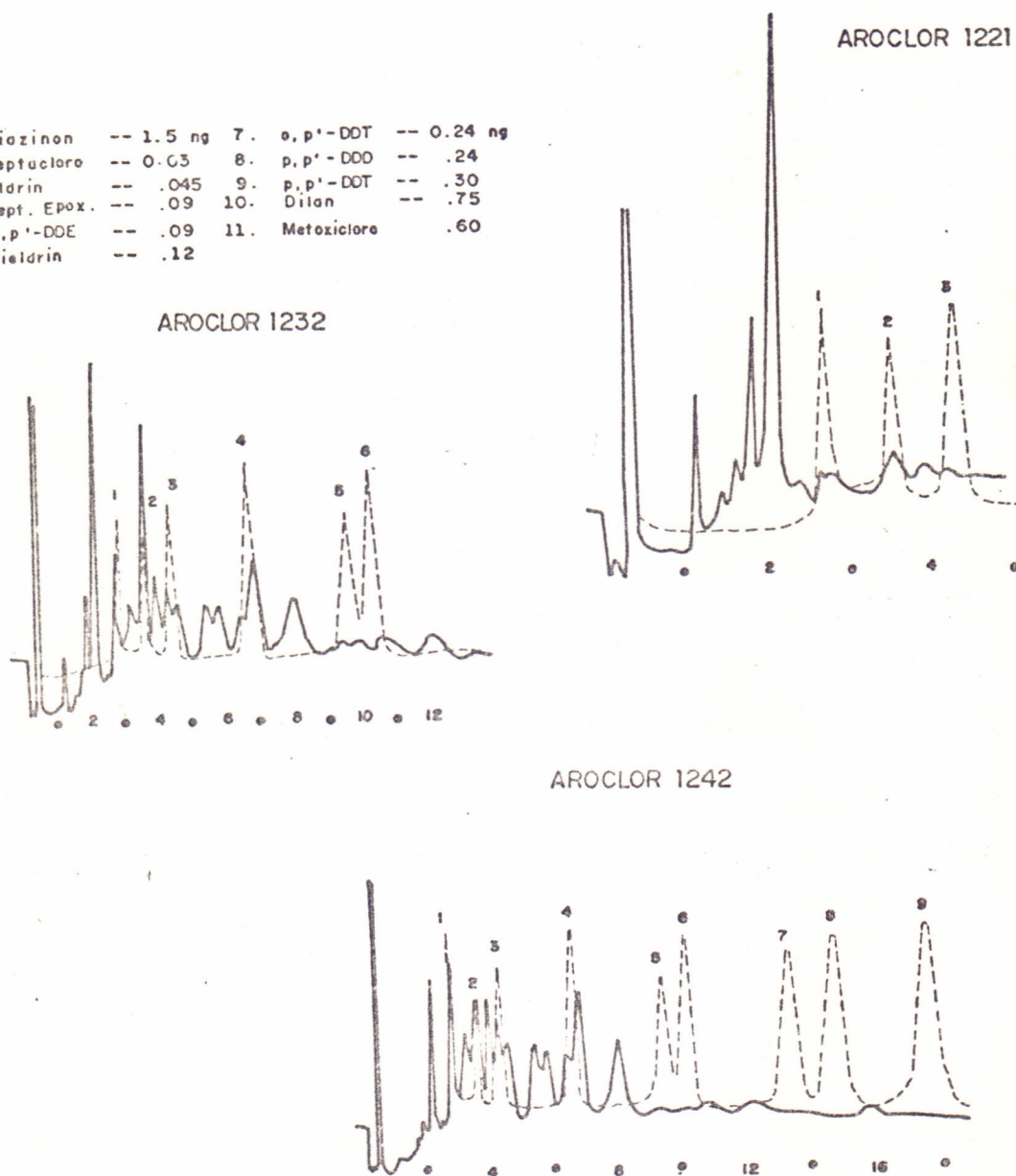
FIGURA 9 - Cromatograma de três PCB's (Aroclor 1221, 1232 e 1242) em coluna de 1,5% de OV-17/1,95% QF-1, nas seguintes condições: Temp. da coluna: 200°C; fluxo do gás de arraste: 60ml/min; detector de ^3\text{H} ; atenuação 10x16. A linha pontilhada mostra uma mistura de pesticidas organoclorados em concentrações de acordo com a figura 55 .
