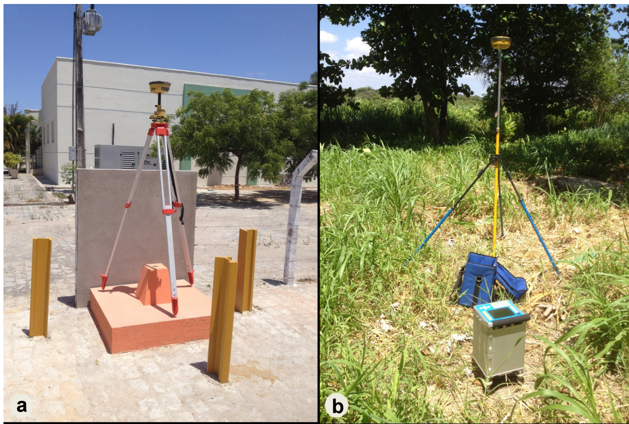
Figura 4: a) Marco gravimétrico do LGPSR/IBGE; e b) Gravímetro e GPS diferencial utilizado no levantamento terrestre e a) Marco gravimétrico do LGPSR/IBGE.
