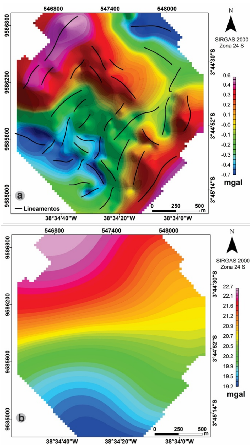
Figura 8: a) Mapa de anomalia Bouguer Regional; b) Mapa de anomalia Bouguer Residual com os lineamentos gravimétricos interpretados.
