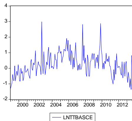
Gráfico D6: Logaritmo natural da balança comercial/termos de troca – setor básicos – do Ceará
