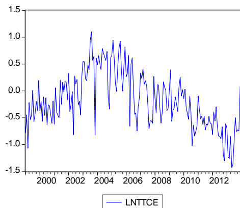
Gráfico D5: Logaritmo natural da balança comercial/termos de troca totais do Ceará (LNTTCE)
