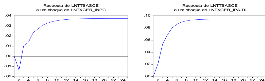
Gráfico 2: Resposta da Balança Comercial dos Básicos a choques na Taxa de Câmbio Fonte: Elaboração Própria a partir do modelo estimado.
