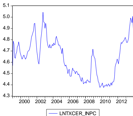
Gráfico D1: Logaritmo natural da taxa de câmbio real efetiva (deflacionado pelo INPC) (LNTXCER_INPC)
