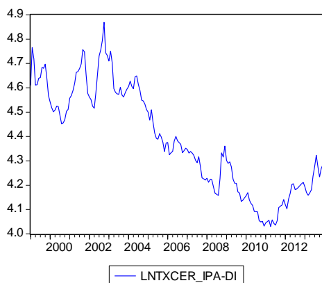
Gráfico D2: Logaritmo natural da taxa de câmbio real efetiva (deflacionado pelo IPA-DI) (LNTXCER_IPA-DI)
