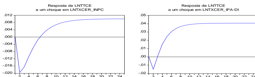
Gráfico 1: Resposta da Balança Comercial Total a choques na Taxa de Câmbio Fonte: Elaboração Própria a partir do modelo estimado.
