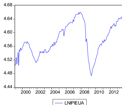
Gráfico D3: Logaritmo natural do índice de produção industrial americano (LNPIEUA)
