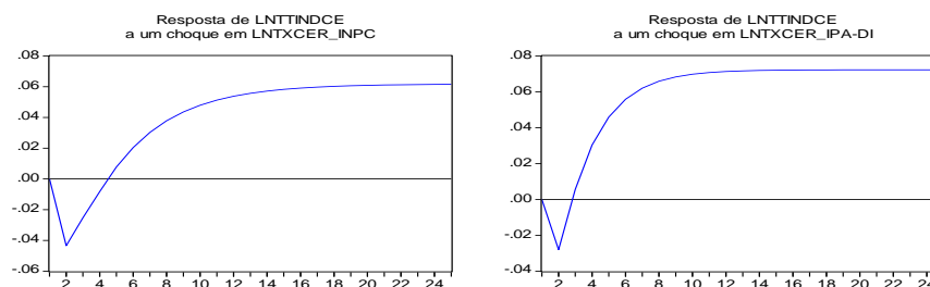
Gráfico 3: Resposta da Balança Comercial Industrializados a choques na Taxa de Câmbio
