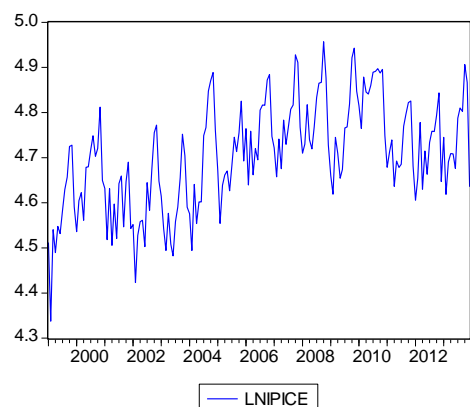
Gráfico D4: Logaritmo natural do índice de produção industrial do Ceará (LNPICE)
