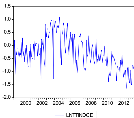
Gráfico D7: Logaritmo natural da balança comercial/termos de troca – setor industrializados – do Ceará (LNTTINDCE)
