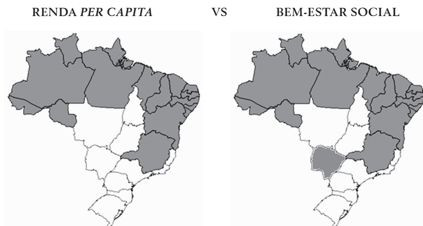
Mapa 1 - Disposição geográfica
