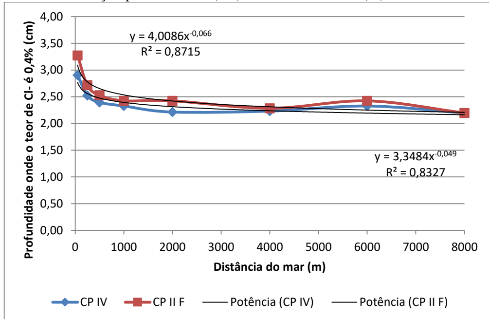
Gráfico 15 - Relação profundidade (cm) e distância ao mar (m) – Praia de Iracema
