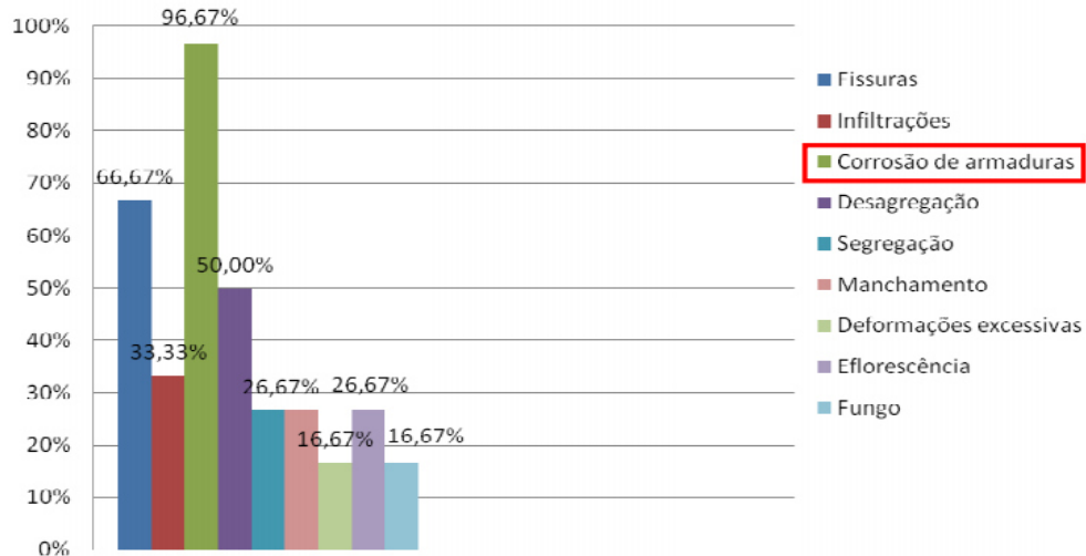
Figura 1 - Manifestações patológicas nas estruturas de concreto
