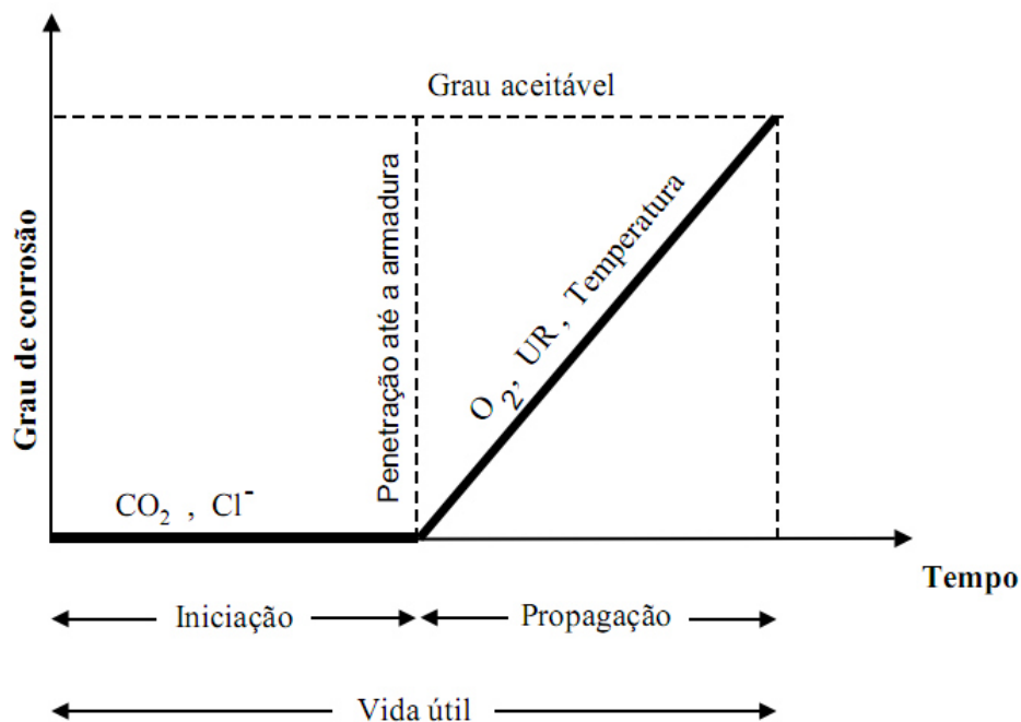
Figura 5 - Modelo de Vida Útil
