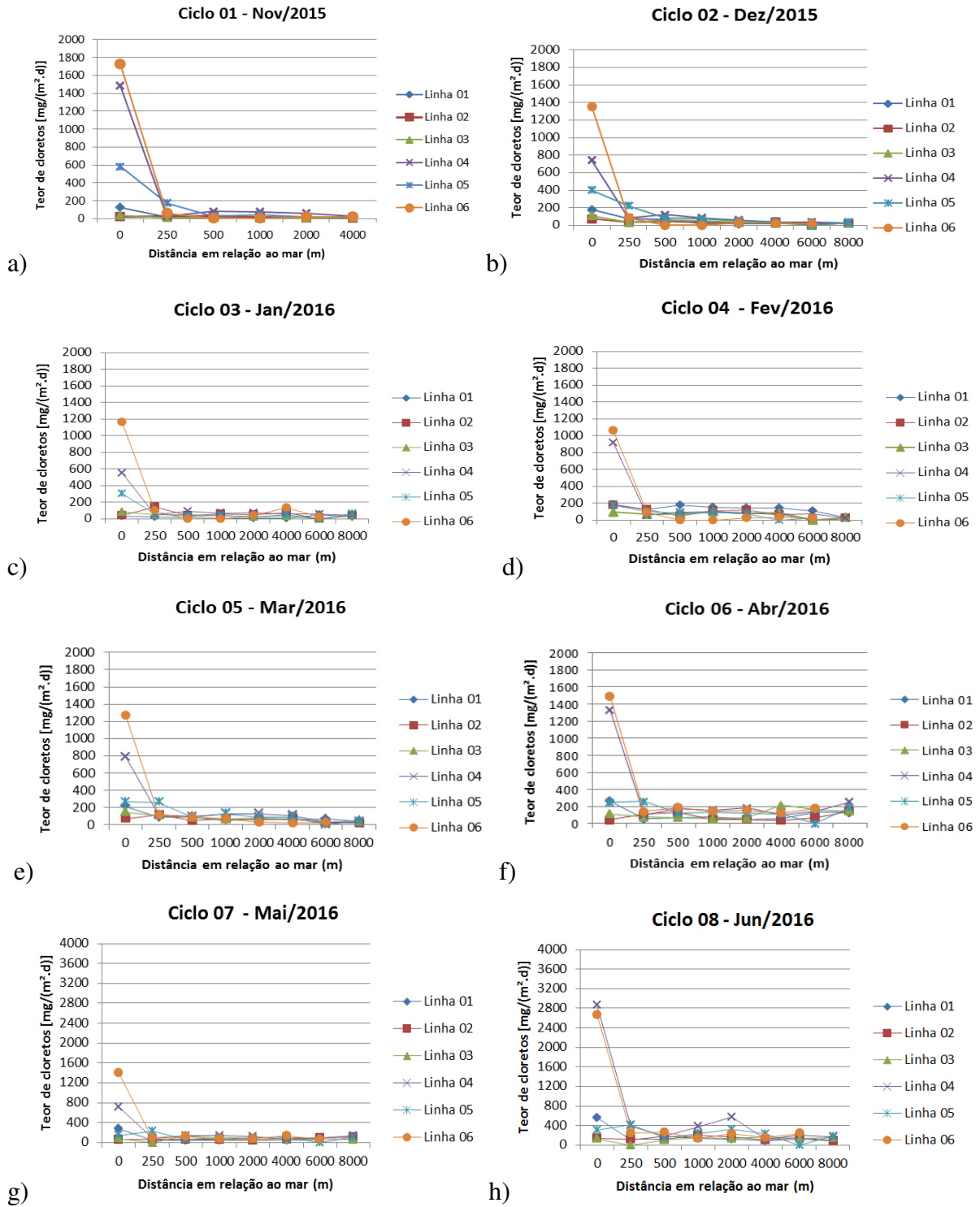
Gráfico 4 - Deposição do Teor de Cloretos [mg/(m 2 .d)] por ciclo
