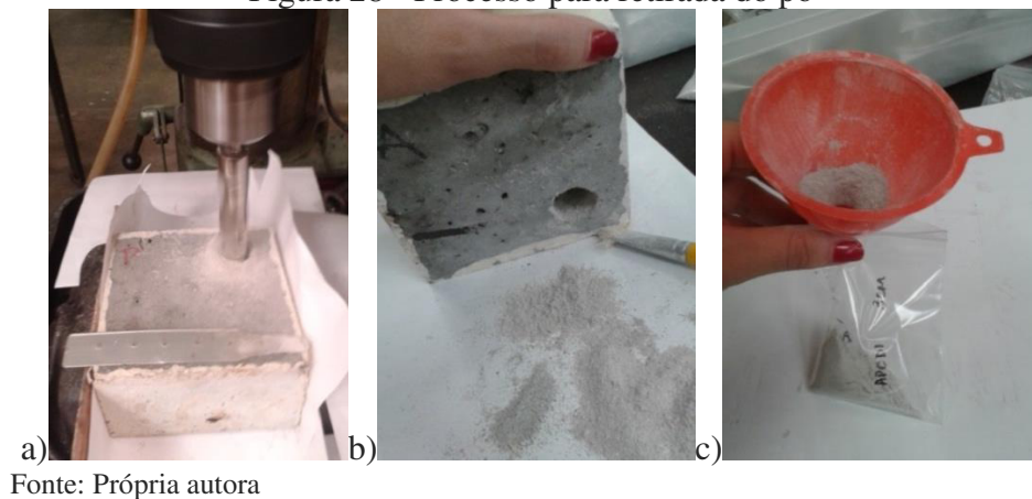
Figura 28 - Processo para retirada do pó
