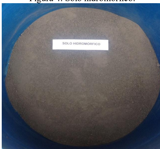
Figura 4: Solo hidromórfico.
