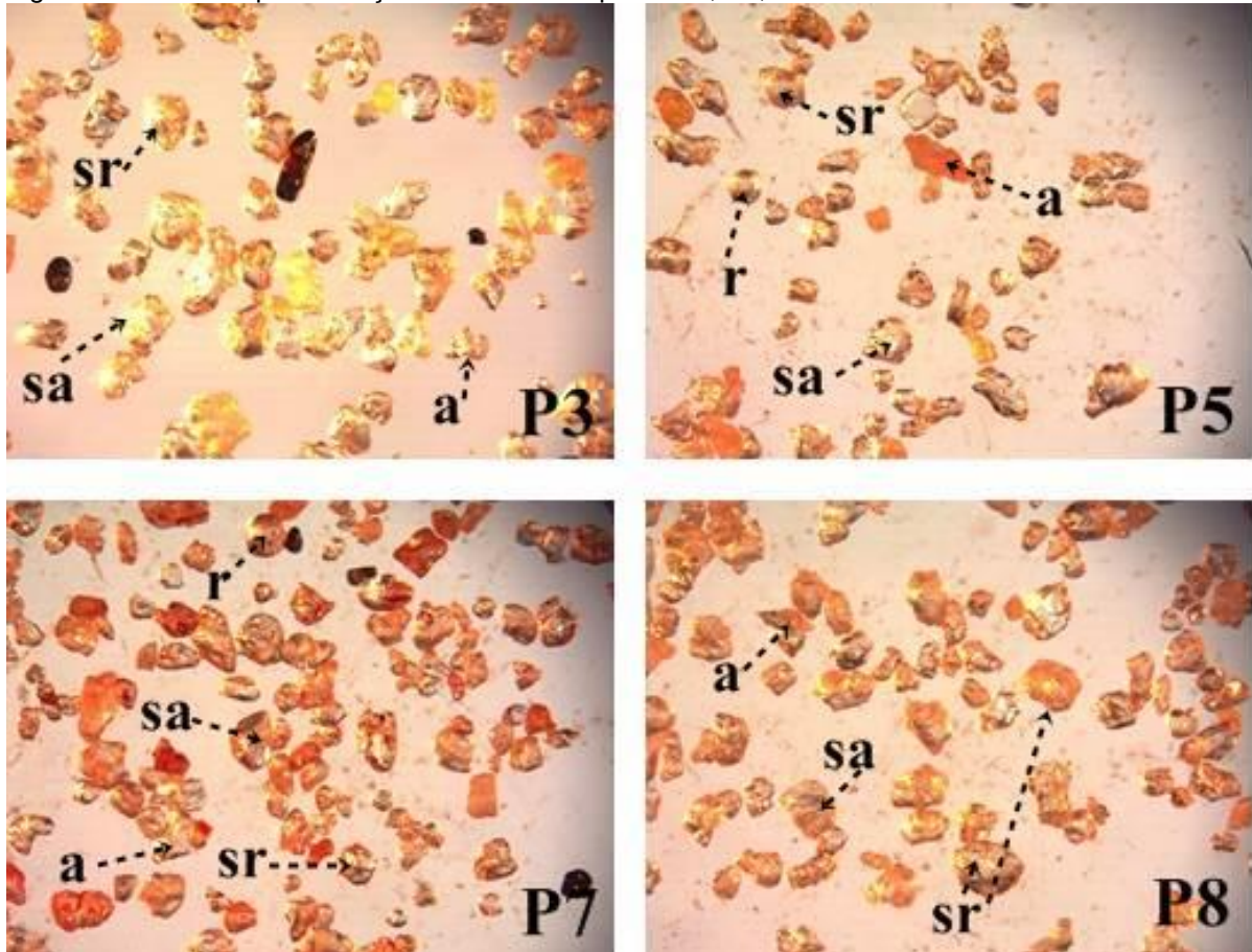
Figura 12- Morfoscopia da fração areia fina dos perfis P3, P5, P7 e P8.
