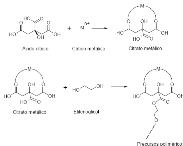
Figura 2 – Representação esquemática do método dos precursores poliméricos modificado.
