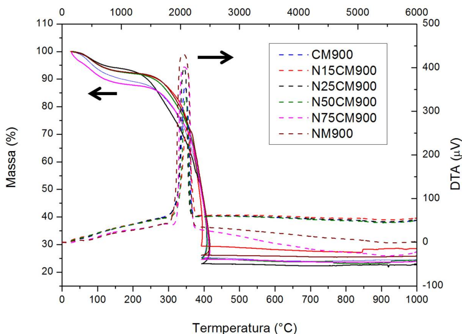
Figura 5 – Análise termogravimétrica (eixo da esquerda e abaixo) e térmica diferencial (eixo da direita e cima) para amostras pré-calcinadas a 250°C.
