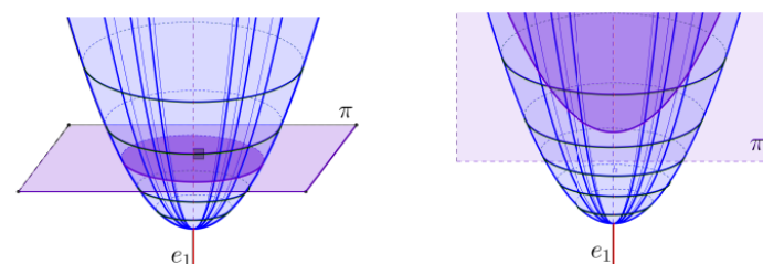
Figura 60 – Parabolóide elíptico
