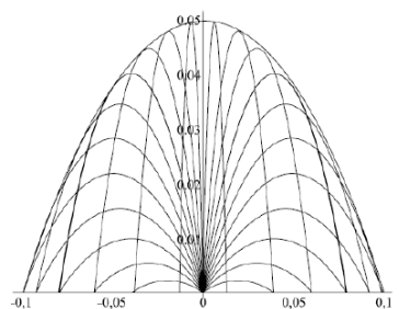
(b) Envoltória a uma família de parábolas
