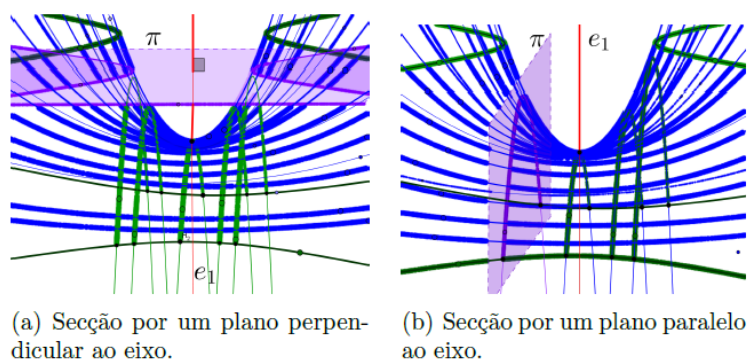
Figura 62 – Parabolóides Hiperbólicos
