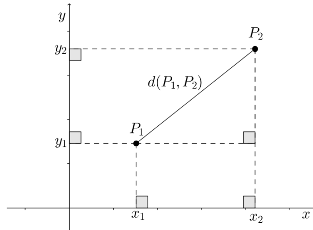
Figura 85 – Distância entre P_1 e P_2 .
