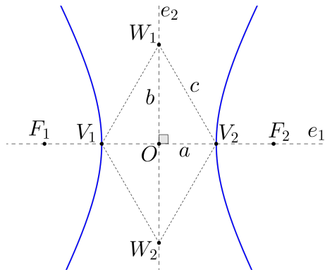
Figura 33 – Triângulos formados com o centro e vértices de uma hipérbole.
