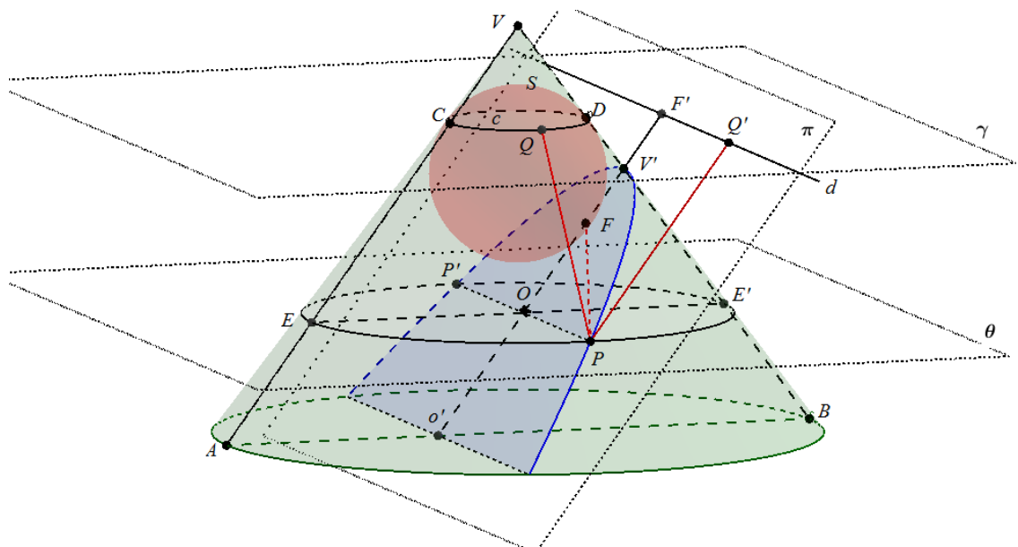
Figura 19 – Parábola no cone de Dandelin
