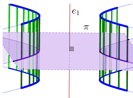
Figura 59 – Cilindro hiperbólico
