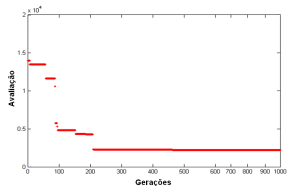
Figura 6. Avaliação da Evolução do Melhor Indivíduo utilizando GA
