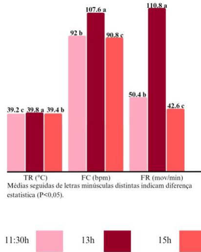
Gráfico 2. Temperatura retal (TR), Frequência cardíaca (FC) e Frequência respiratória (FR) de carneiros Somalis expostos a radiação solar direta.
