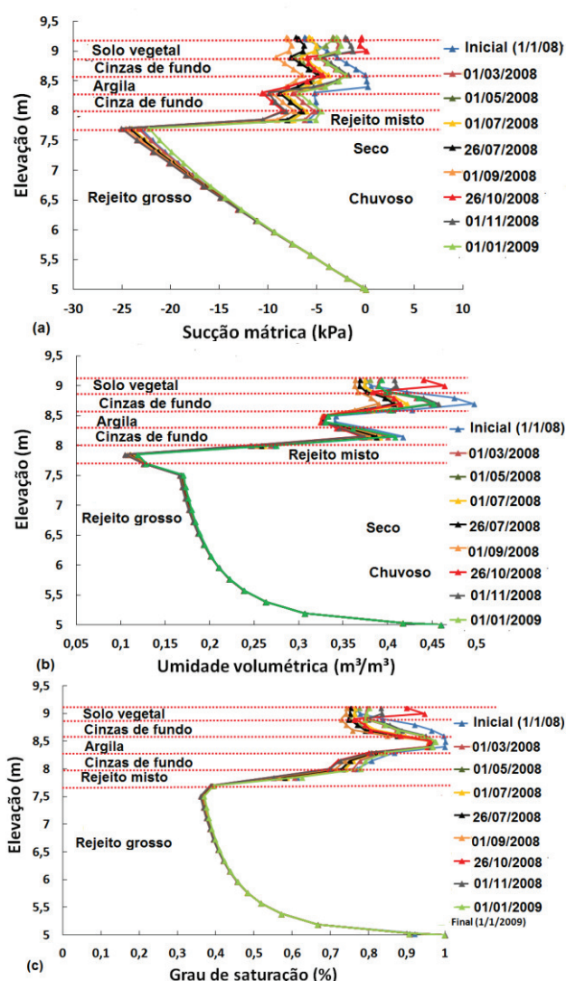
Figura 6. Perfis: (a) sucção, (b) umidade vol. e (c) grau de saturação com o tempo e a profundidade no modelo CS2.
