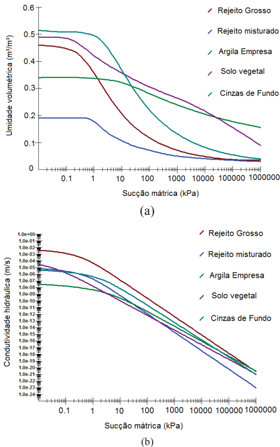
Figura 2. (a) Curvas de retenção e (b) condutividade não saturada dos materiais.
