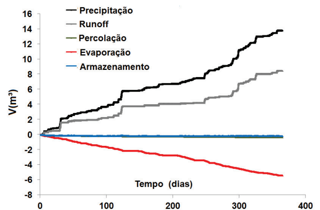
Figura 5. Parcelas do balanço hídrico no modelo CS1.
