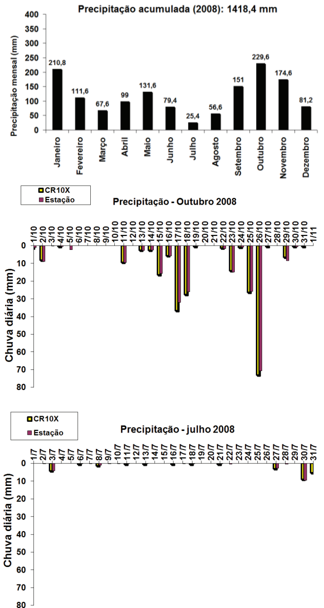
Figura 3. Dados de precipitação em 2008.
