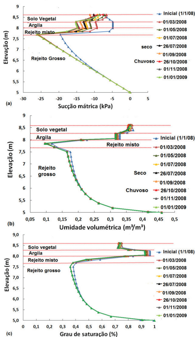
Figura 4. Perfis: (a) sucção, (b) umidade vol. e (c) grau de saturação com o tempo e a profundidade no modelo CS1.
