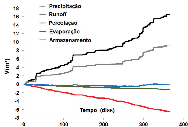
Figura 7. Parcelas do balanço hídrico no modelo CS2.
