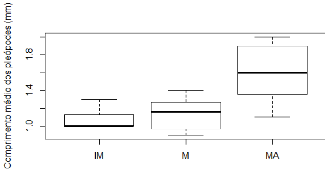
Figura 9 – Fêmeas de Clibanarius sclopetarius . Boxplot com o comprimento médio dos pleópodes para cada estágio de maturação.
