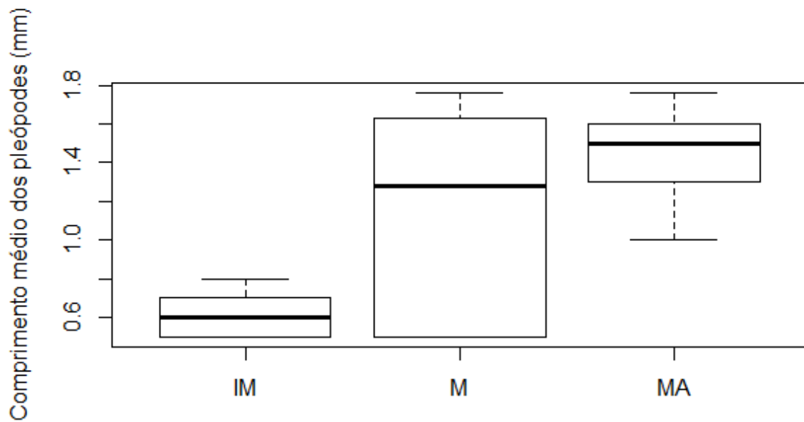
Figura 8 – Fêmeas de Clibanarius sclopetarius . Boxplot com o comprimento médio dos pleópodes para cada estágio de maturação.
