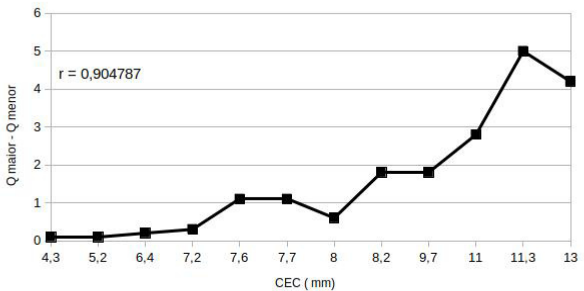
Figura 11 – (Correlação entre Comprimento do escudo cefálico (CEC) e diferença entre quelípodo maior e menor (Q maior - Q menor) em indivíduos de Clibanarius sclopetarius .
