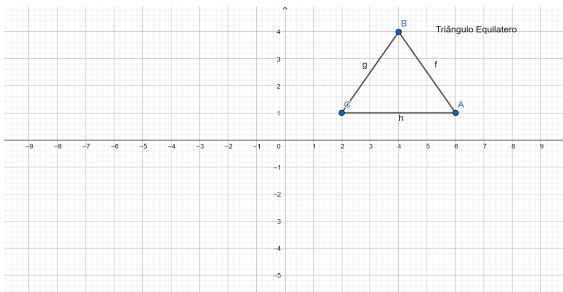
Figura 1 – Triângulo Equilátero
