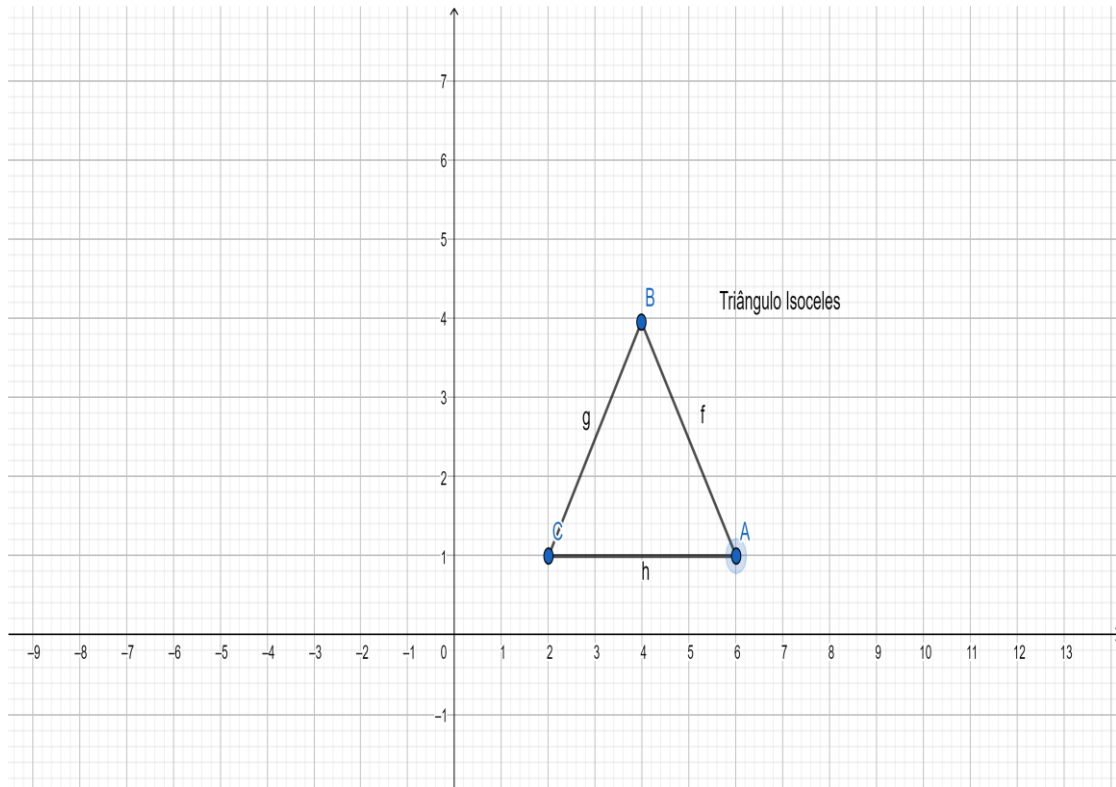
Figura 2 – Triângulo Isósceles
