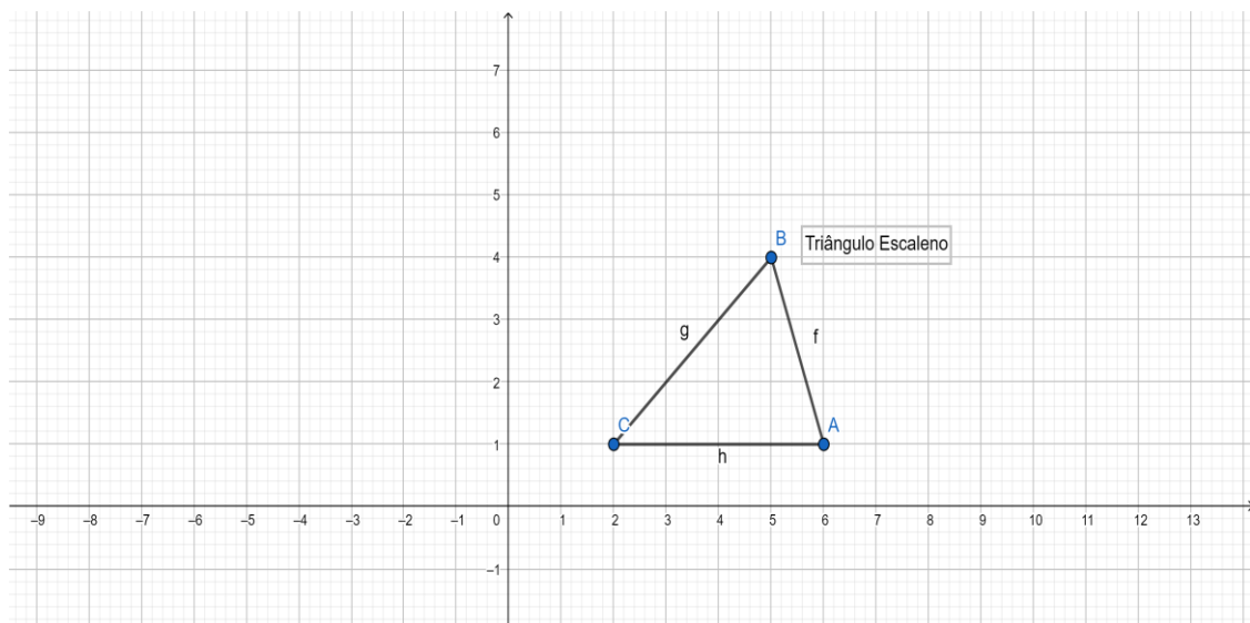
Figura 3 – Triângulo Escaleno
