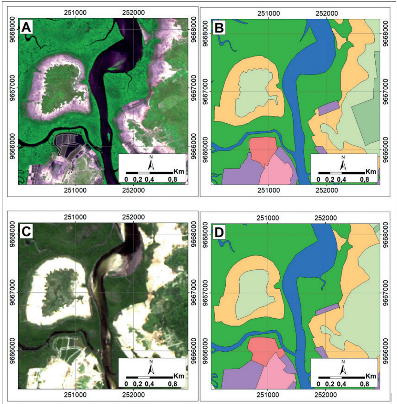
Figura 2 A. Análise comparativa multitemporal da imagem RapidEye de 2012 usando 3R5G2B; B. Identificação das unidades do uso e cobertura da terra referente a 2012; C. Da imagem Landsat 8 de 2015 usando 3R4G2B8I; D. Identificação das unidades do uso e cobertura da terra 2015.
