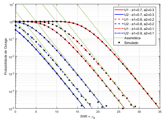
Fig. 2. Probabilidade de outage vs SNR para M = 3 e N = 3 , d_{SR} = 0.5 , d_1 = 1.5 e d_2 = 0.5 .
