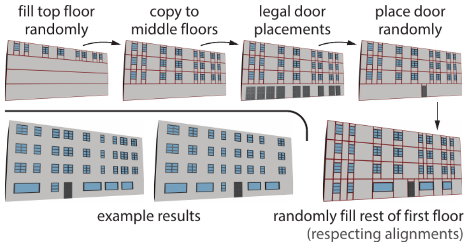
Figura 14 – Modelos de fachadas com elementos e alinhamentos aleatórios. Acima: abordagem de solução geral, na qual as linhas de divisão são mostradas em vermelho. Abaixo: exemplo de resultados para diferentes parâmetros.
