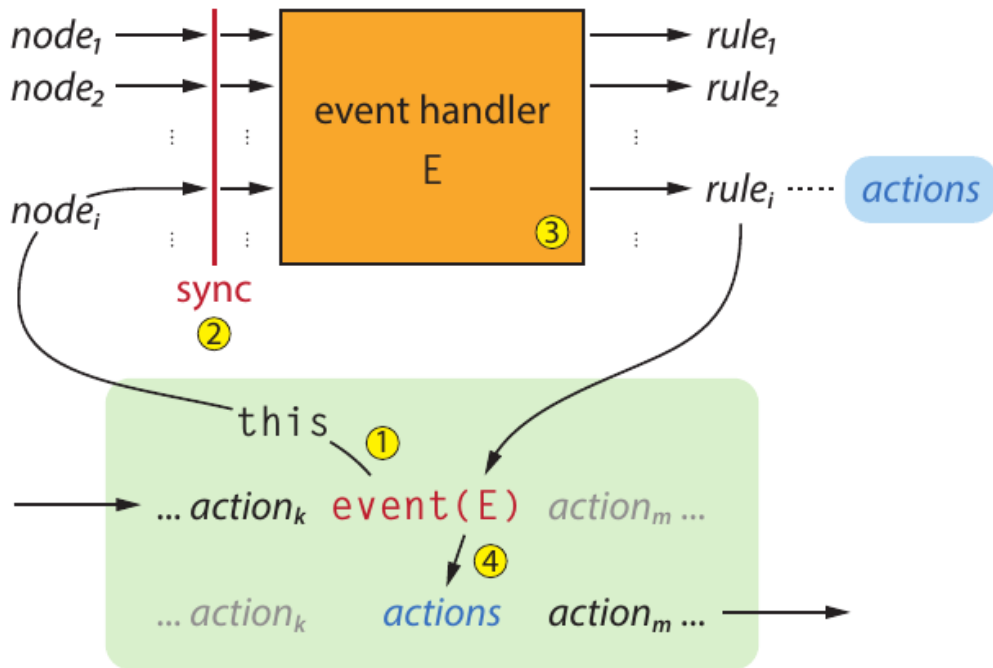
Figura 11 – Representação do manipulador de eventos.
