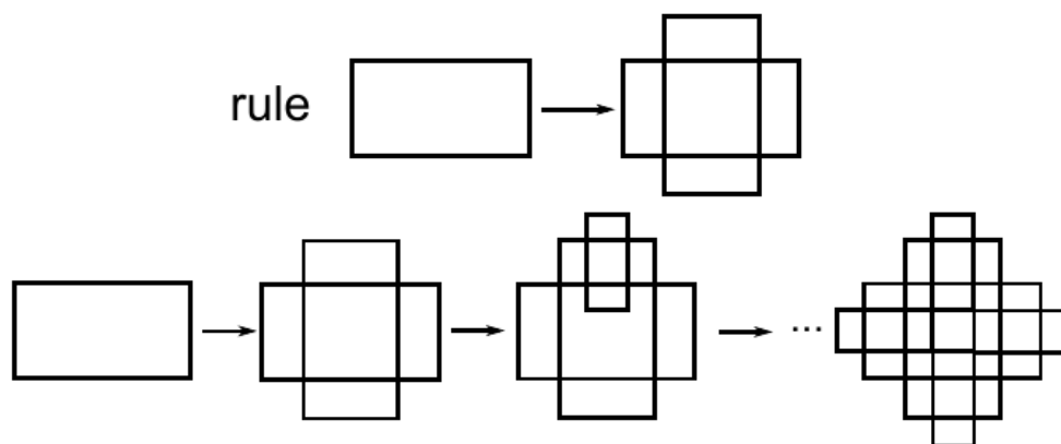
Figura 80 – Gramática para gerar planta de igreja na forma de cruz grega.
