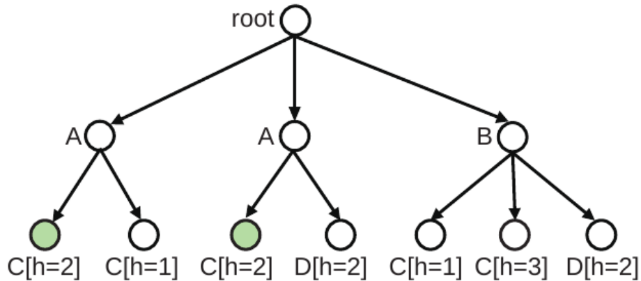
Figura 21 – Grafo abstrato da seleção de nós.
