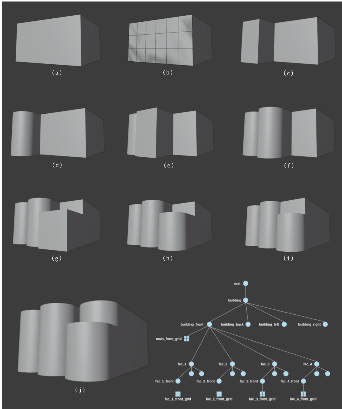
Figura 66 – Modelo de massa do edifício da Figura 49.
