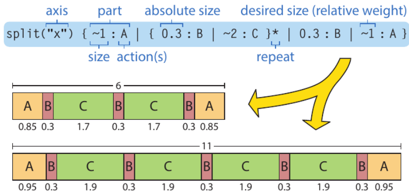
Figura 15 – Exemplo de operação split , mostrando o resultado para diferentes valores de entrada, neste caso, 6 e 11.
