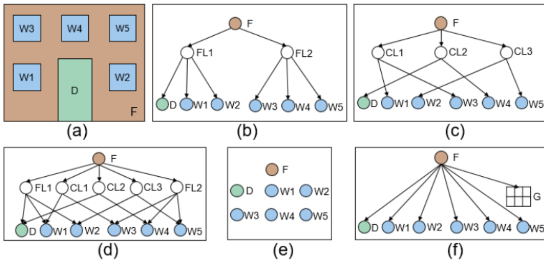
Figura 18 – As ilustrações (b), (c), (d), (e) e (f), representam diferentes perspectivas da árvore de formas em relação ao design da fachada (a).
