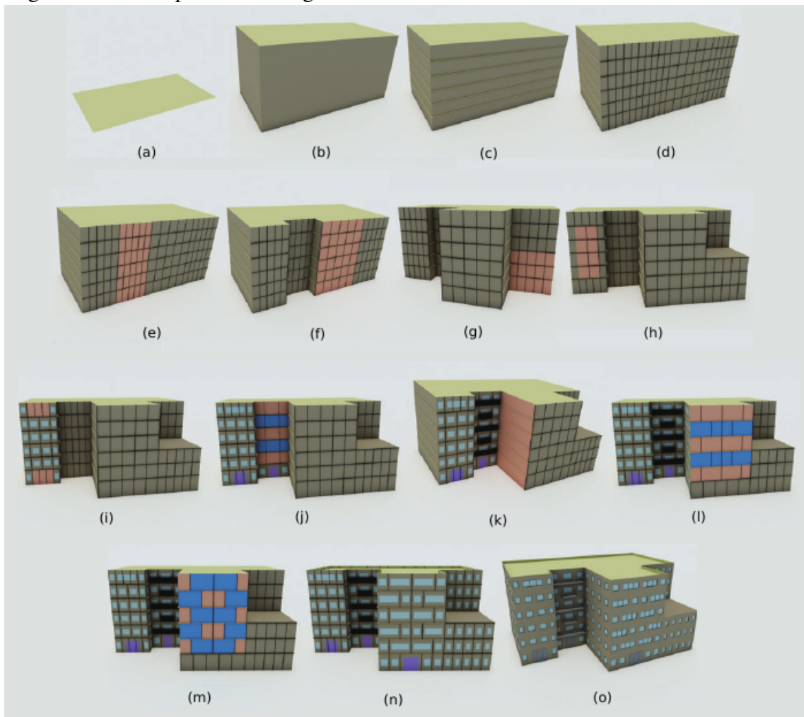
Figura 29 – Exemplo de modelagem utilizando SELEX .
