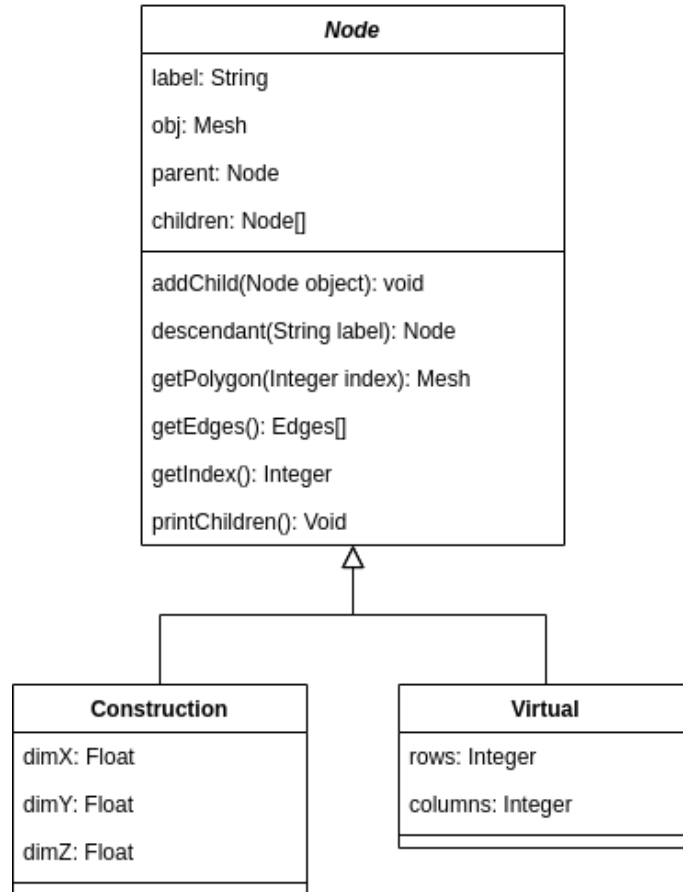
Figura 54 – Diagrama de classes referente à estrutura da árvore de formas.
