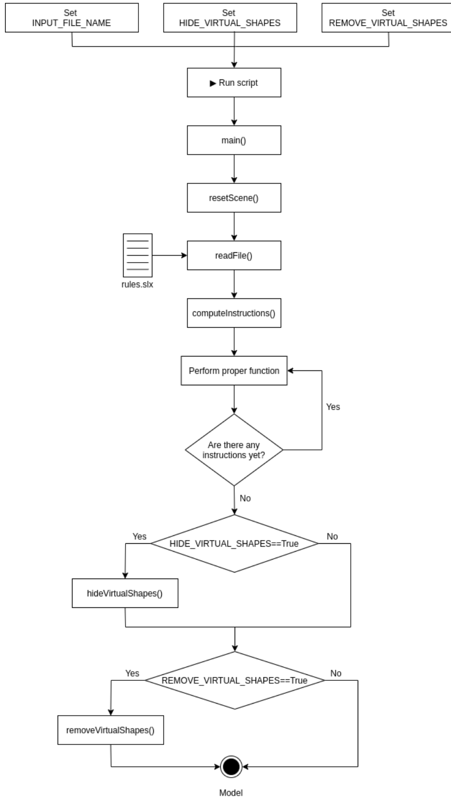
Figura 53 – Fluxograma de execução.
