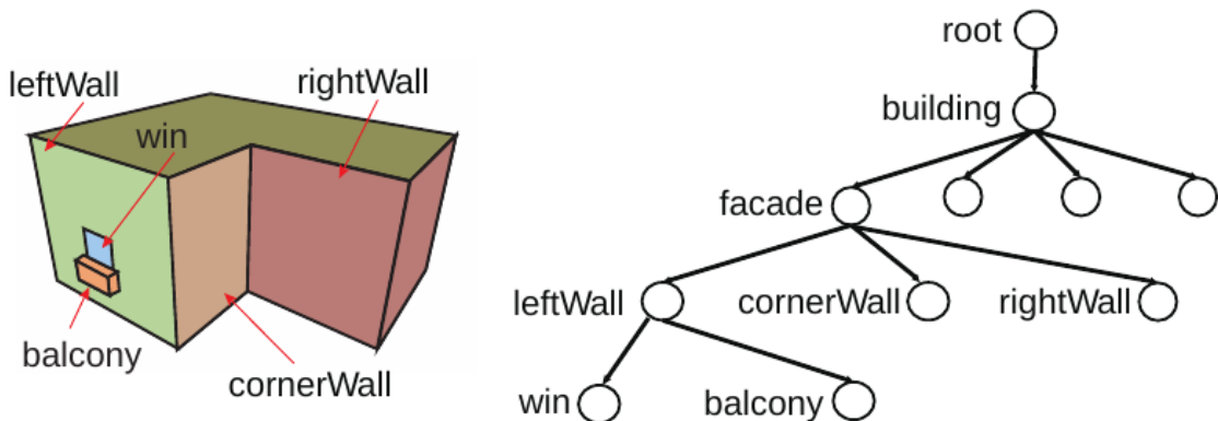
Figura 19 – Para a forma atual ( leftWall ), é demonstrada uma forma contida ( win ), uma forma anexada ( balcony ) e uma forma conectada ( cornerWall ).
