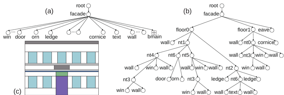
Figura 27 – Exemplo da árvore de formas gerada pela SELEX em (a), e pela CGA Shape em (b), com base na fachada (c).
