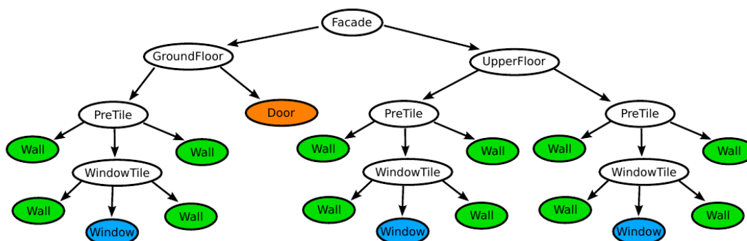
Figura 84 – Árvore de derivação referente à fachada representada na Figura 85.
