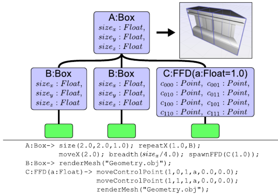
Figura 38 – Aplicação de regras de modelagem da G^2 .
