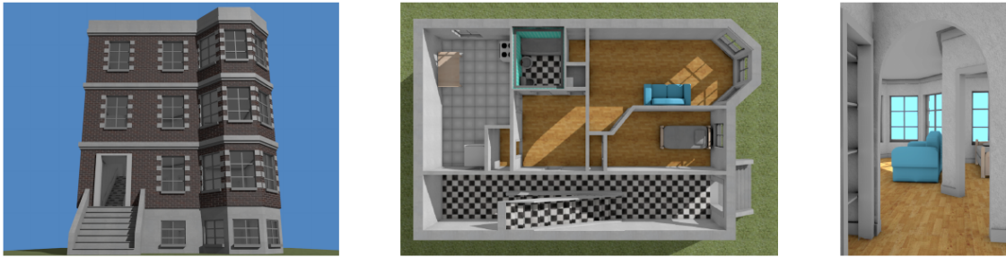
Figura 3 – Modelo de uma casa (à esquerda), com vista superior do primeiro andar (ao centro) e vista de dentro (à direita).
