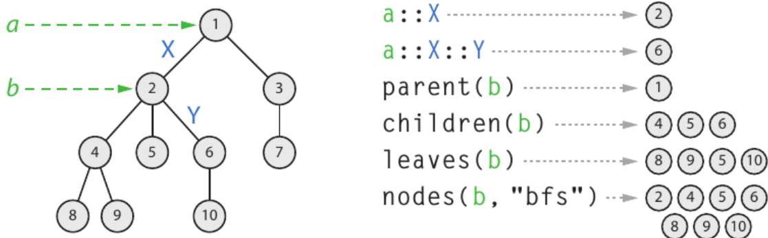
Figura 9 – Opções de navegação na árvore. Neste caso, a e b são valores representando as formas dos nós 1 e 2, respectivamente, enquanto X e Y são rótulos.
