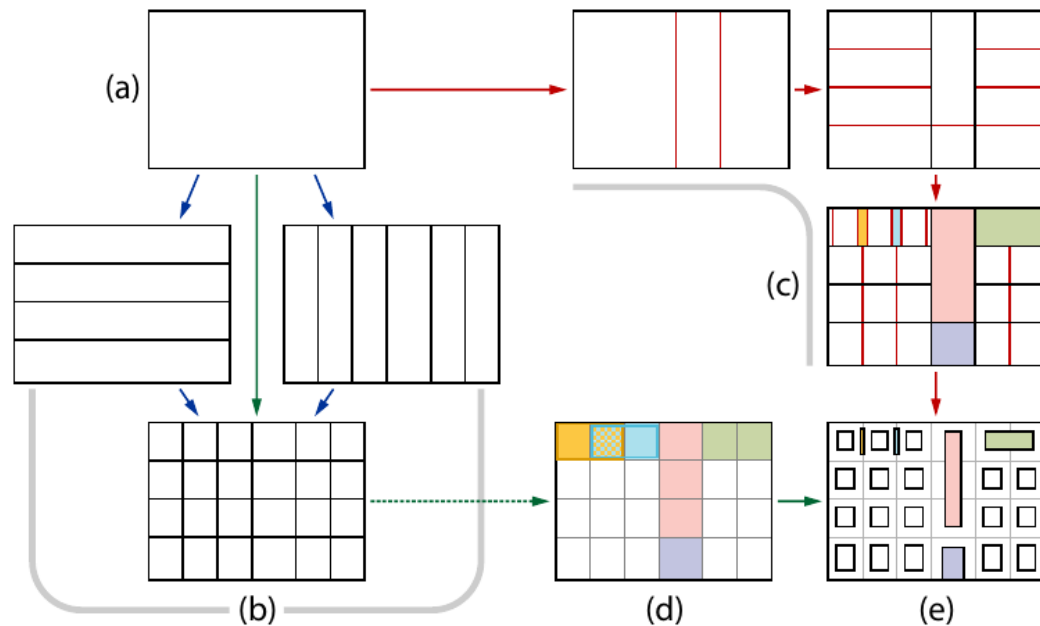
Figura 17 – Ilustração dos paradigmas de modelagem SELEX e CGA Shape .
