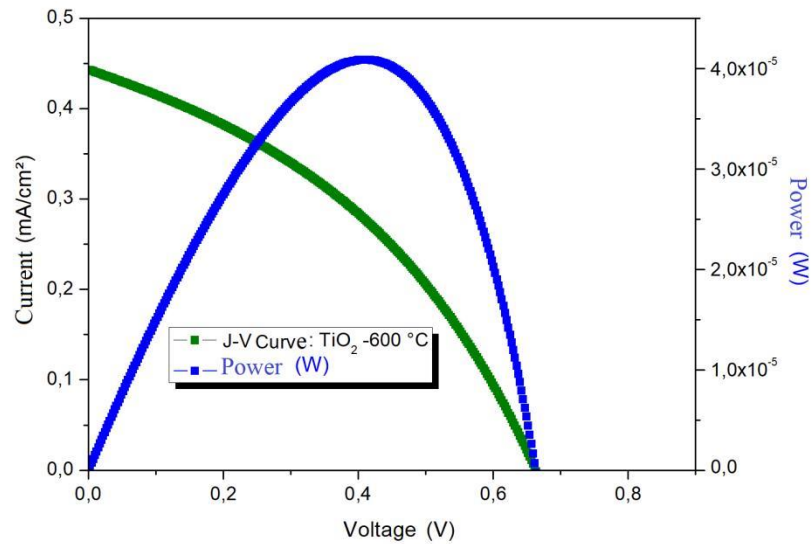
Figura 10: Curva J-V da amostra 600.
