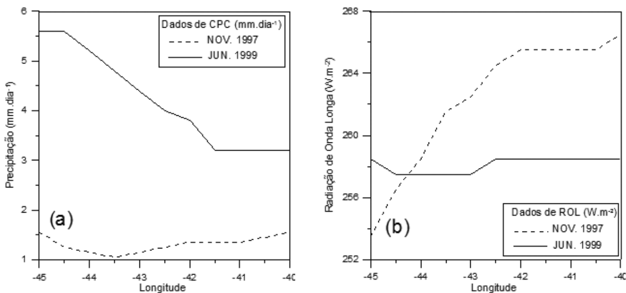
Figura 4 – (a) Dados de precipitação (mm.dia -1 ) fornecido pelo CPC – Climate Prediction Center, USA, e (b) dados de OLR – Outgoing Longwave Radiator (W.m -2 ), obtidos durante os dois períodos de coletas hidrográficas do Programa REVIZEE/N (Novembro/1997 e Junho 1999).
