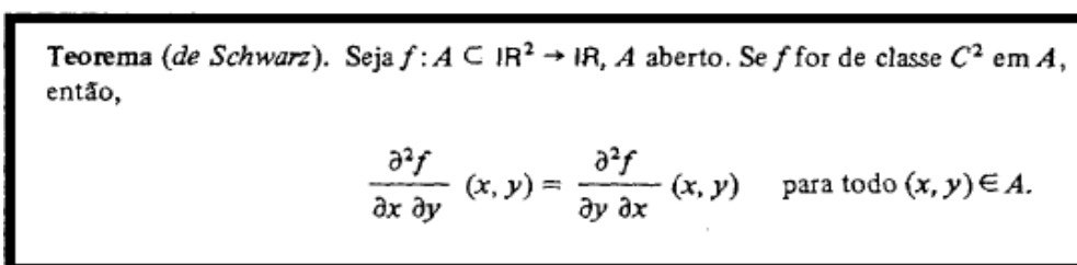
FIGURA 7. Descrição do teorema de Clairaut-Schwarz descrito em Guidorizzi (2001). FONTE: Guidorizzi (2010, p. 276).
