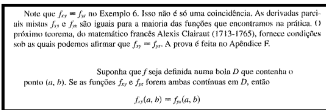
FIGURA 6. Descrição do teorema de Clairaut-Schwarz descrito em Stewart (2001b). FONTE: Stewart (2001b).
