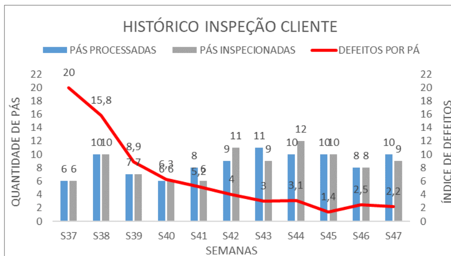
Gráfico 11 – Média de defeitos por pá por semana – Inspeção do Cliente S47
