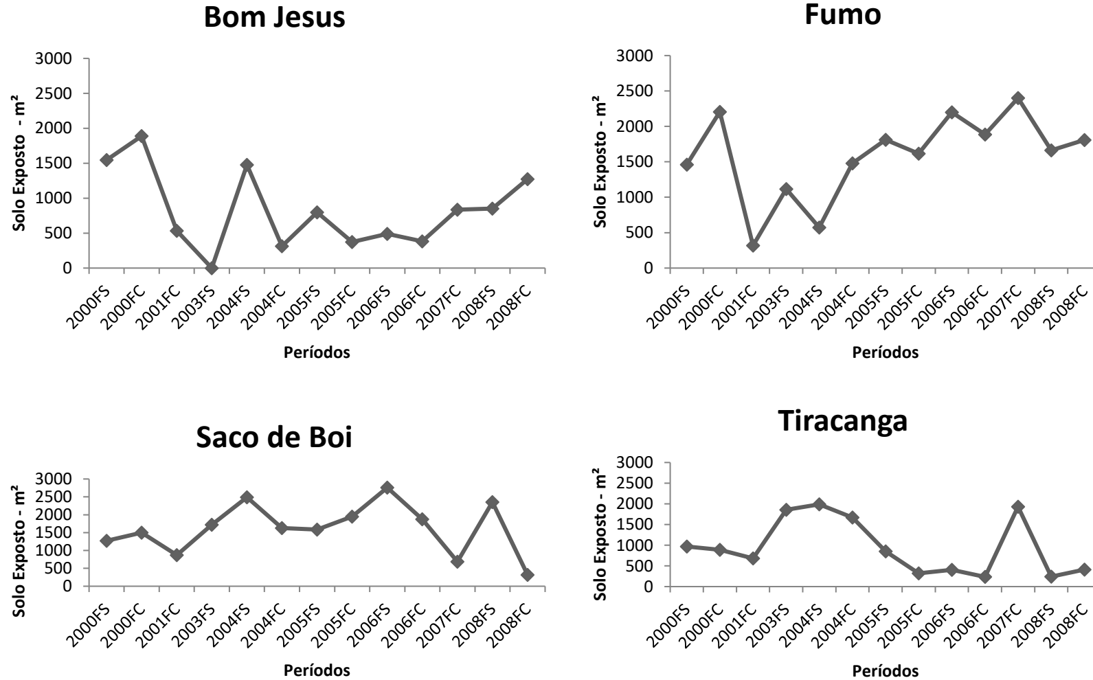
Figura 25 - Área de solo exposto nos períodos secos e chuvosos ao longo dos anos de 2000 a 2008
