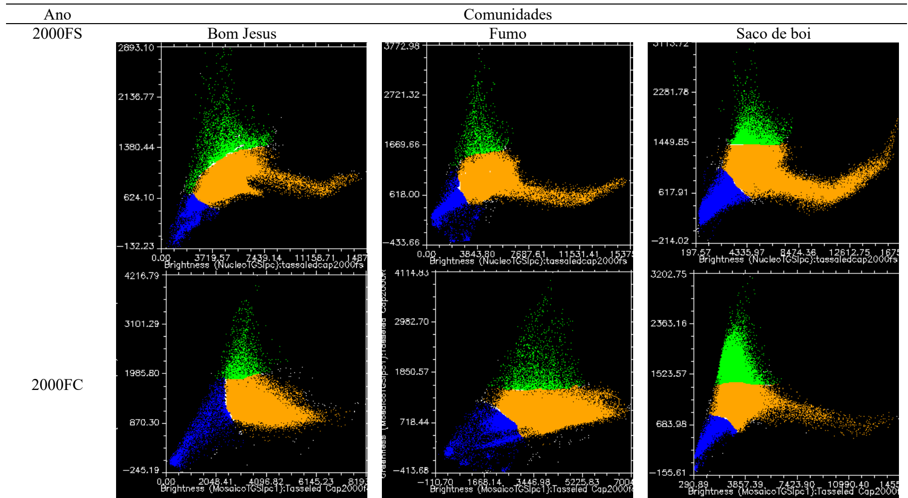
Figura 31 - Brightness e Greenness paras as comunidades Bom Jesus, Fumo e Saco de boi
