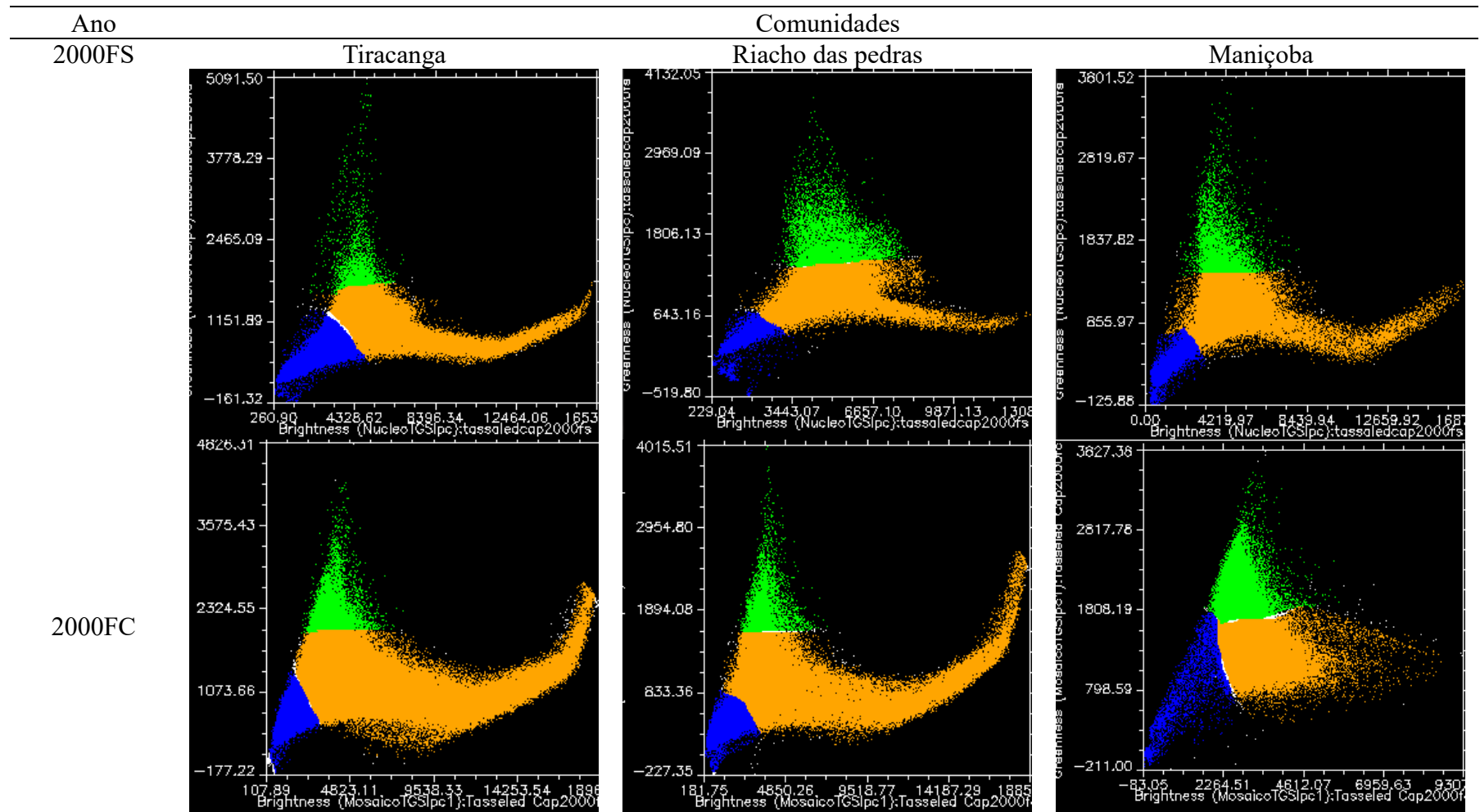
Figura 32 - Brightness e Greenness paras as comunidades Tiracanga, Riacho das pedras e Maniçoba
