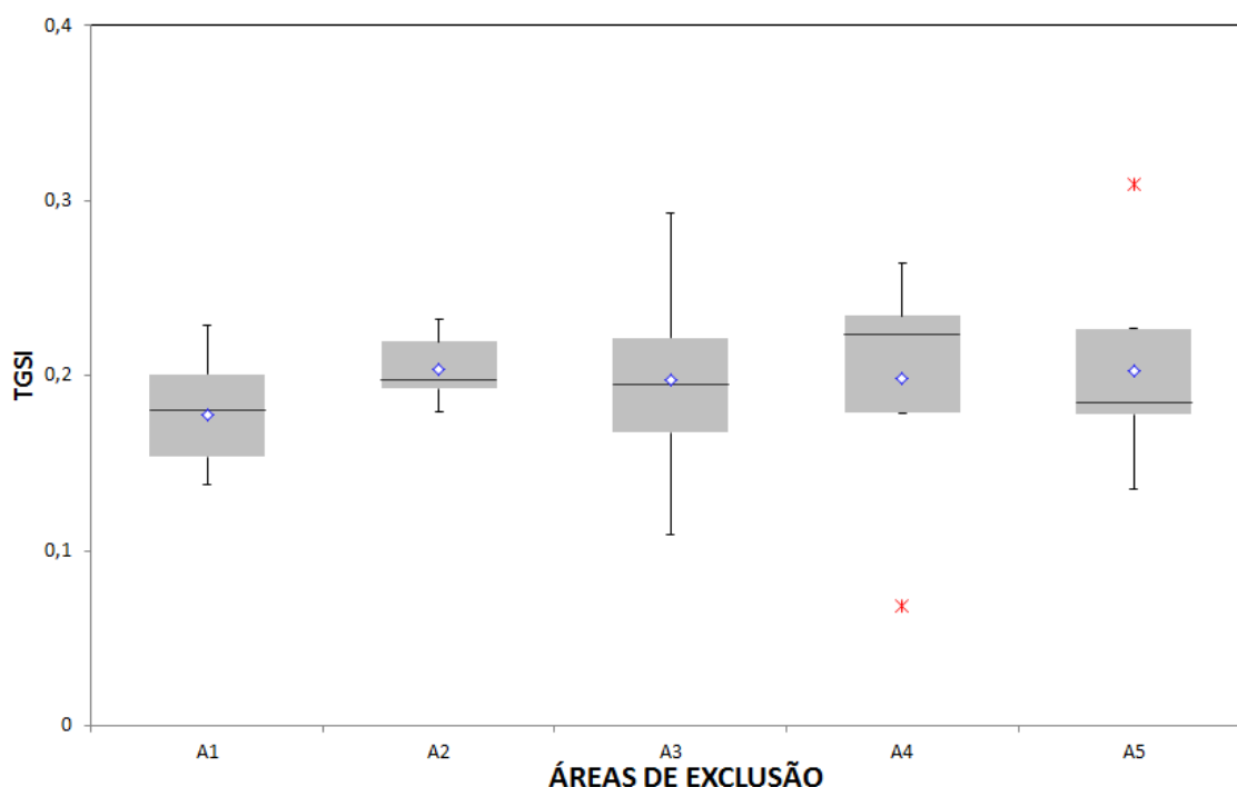
Figura 16 - Box Plot de dados de TGSi para as áreas de exclusão
