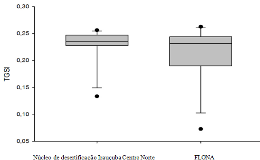
Figura 15 - Box Plot de dados de TGSi para as áreas desertificadas e preservadas
