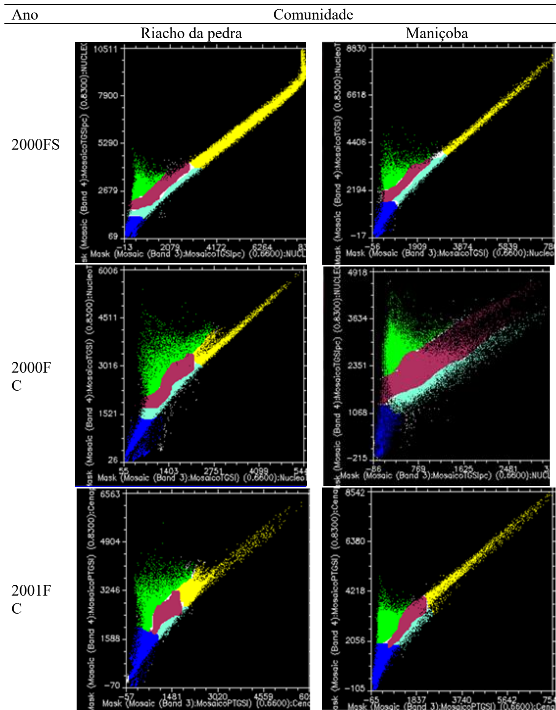
Figura 24 - Linha de solo para as comunidades Maniçoba e Riacho da pedra
