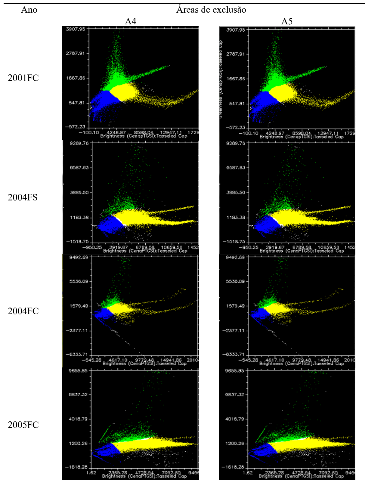
Figura 41 - Plano de vegetação de áreas de exclusão A4 e A5 entre os anos de 2000 a 2008
