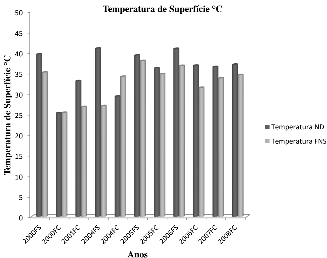
Figura 48 - Temperatura de Superfície do Núcleo e do FLONA
