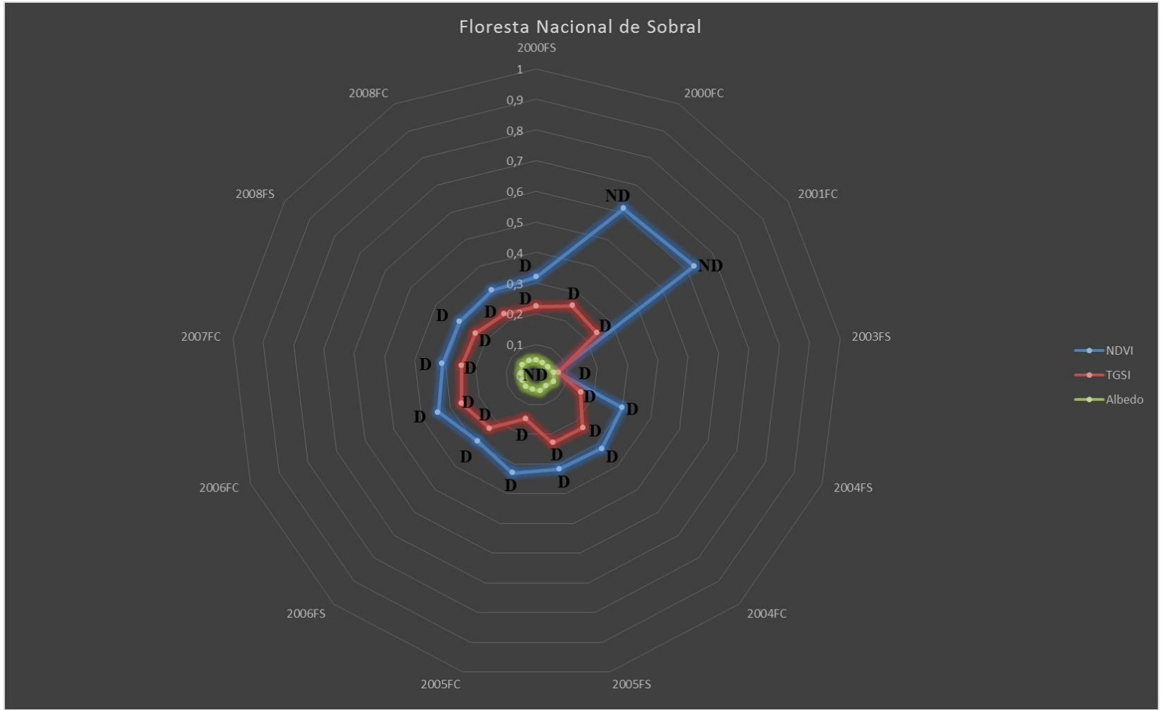
Figura 46 - NDVI, TGSi e Albedo para FLONA entre os anos de 2000 a 2008
