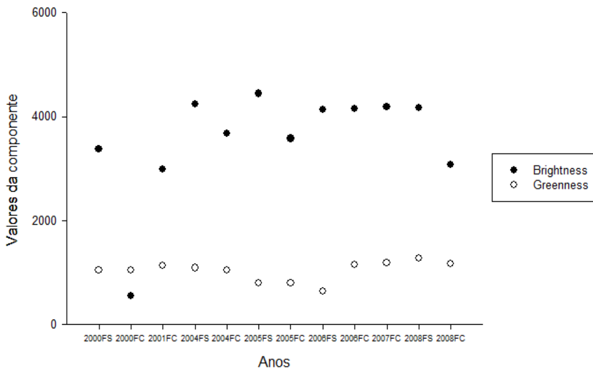
Figura 35 - Valores de Brightness e Greenness FLONA
