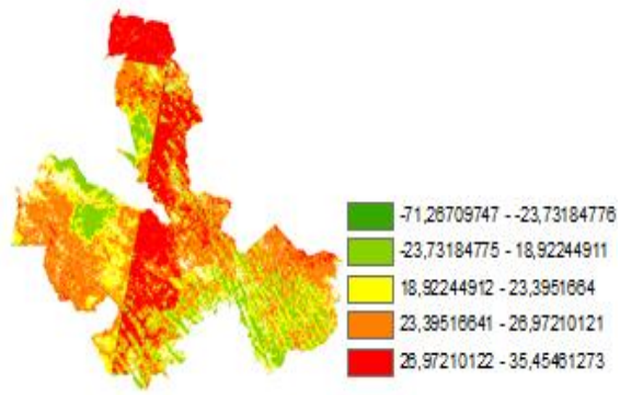
Figura 42 - Mapas de Temperatura de Superfície (°C) para o Núcleo de Desertificação Irauçuba Centro Norte
