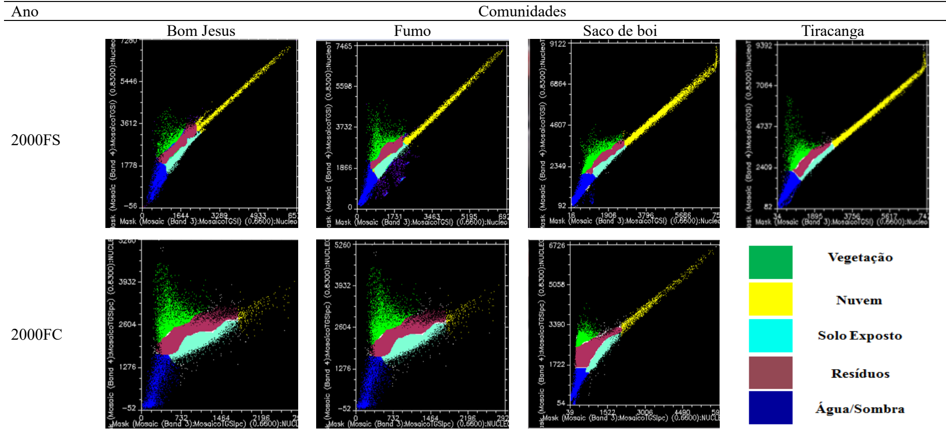
Figura 23 - Linha de solo para as comunidades Bom Jesus, Fumo, Saco de boi e Tiracanga
