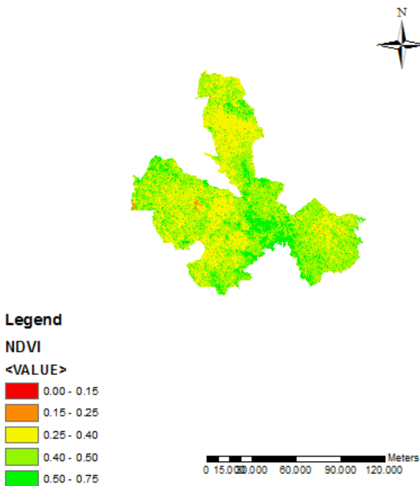
Figura 49 - Pixels de NDVI entre os anos de 2000 a 2008 no núcleo
