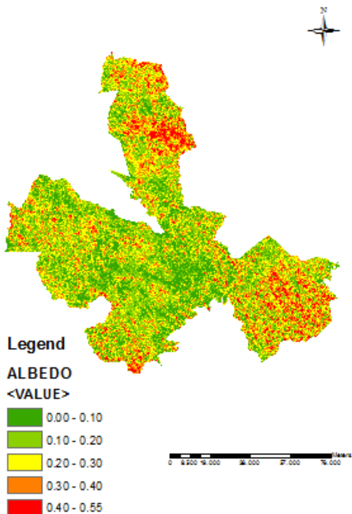
Figura 51 – Pixels de Albedo de 2000 a 2008 no núcleo de desertificação
