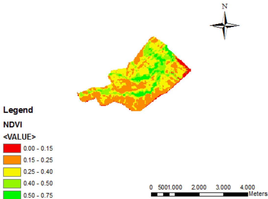
Figura 50 - Pixels de NDVI constantes durante os anos de 2000 a 2008 no FLONA
