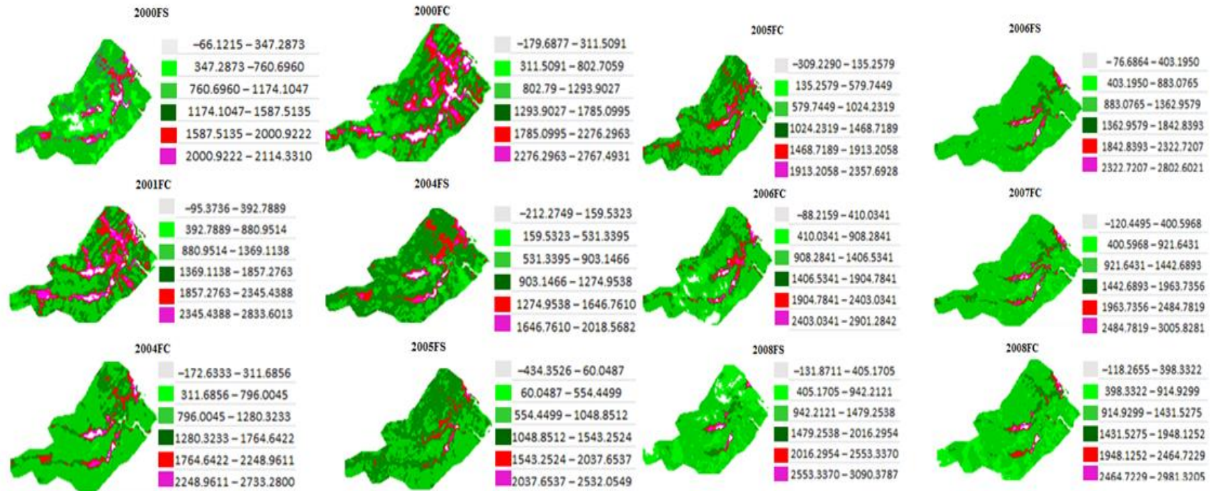
Figura 37 - Mapas de Greenness para FLONA durante os períodos secos e chuvosos entre os anos de 2000 a 2008
