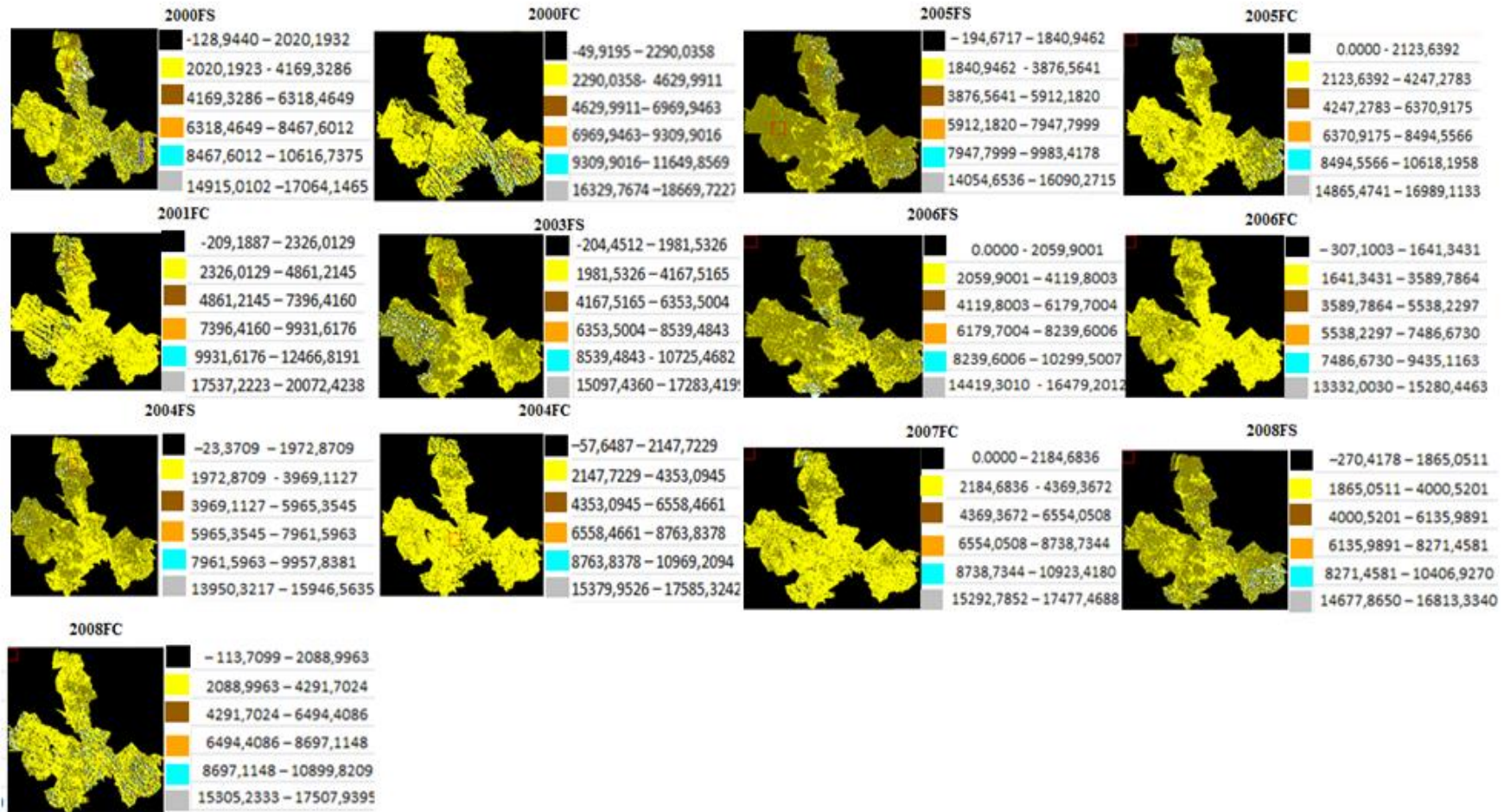
Figura 33 - Mapas de Brightness para o núcleo de desertificação Irauçuba Centro Norte durante os períodos secos e chuvosos entre os anos de 2000 a 2008
