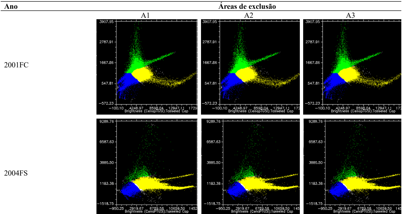
Figura 40 - Plano de vegetação de áreas de exclusão A1, A2 e A3 entre os anos de 2000 a 2008
