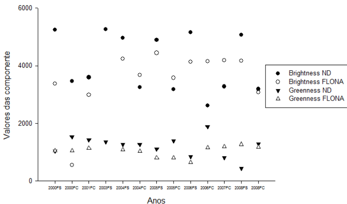
Figura 47 - Brightness e Greenness no núcleo e no FLONA
