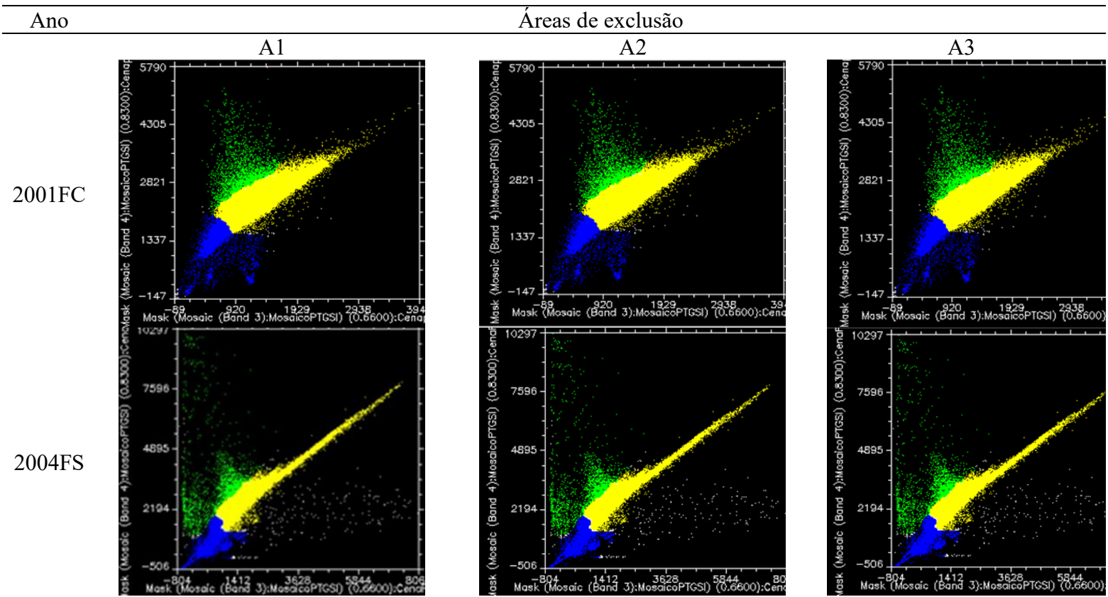
Figura 28 - Linha de solo para as áreas de exclusão A1,A2 e A3
