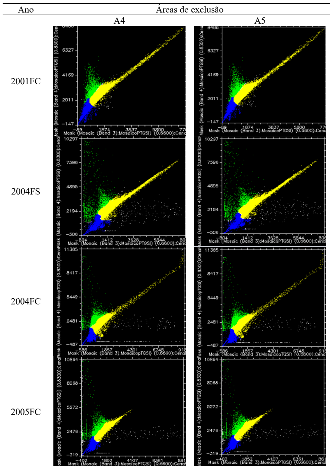
Figura 29 - Linha de solo para as áreas de exclusão A4 e A5
