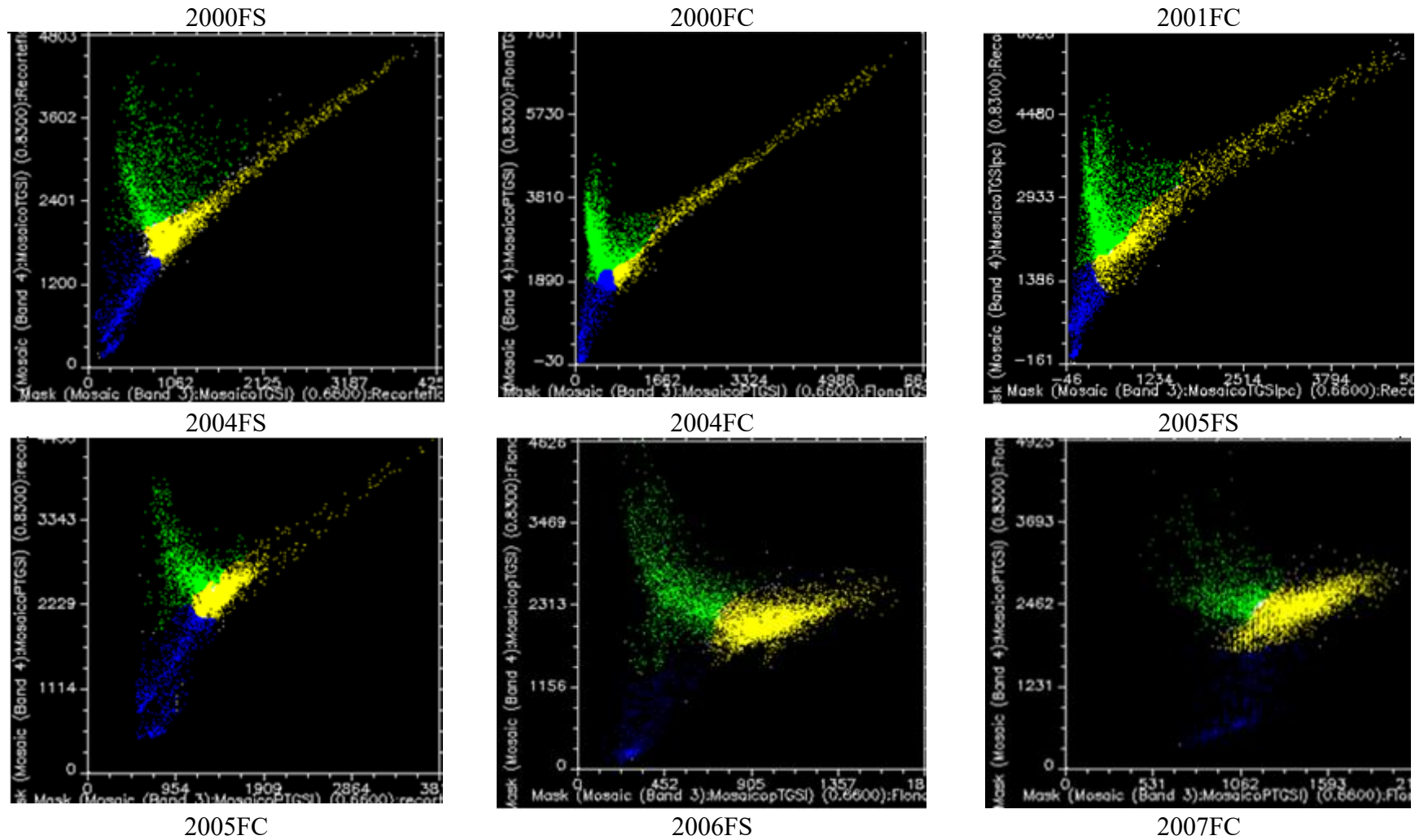
Figura 27 - Linha de Solo para FLONA nos períodos secos e chuvosos ao longo dos anos de 2000 a 2008
