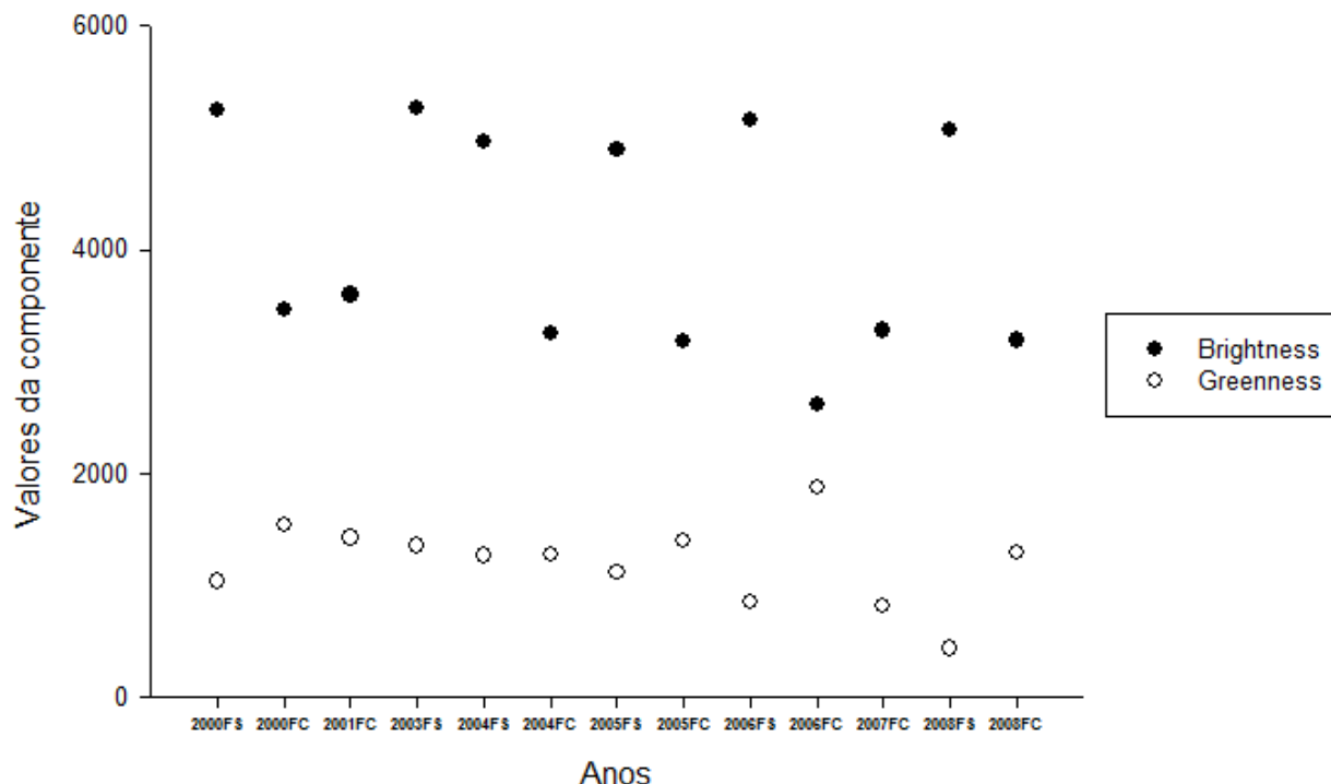
Figura 30 - Brightness e Greenness no Núcleo
