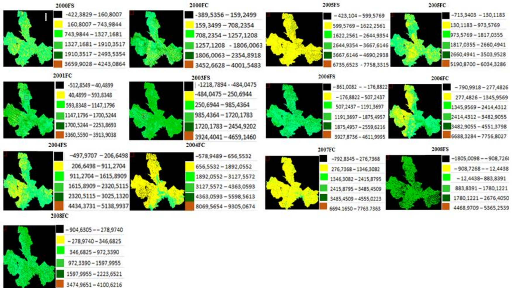
Figura 34 - Mapas de Greenness para o núcleo de desertificação Irauçuba Centro Norte durante os períodos secos e chuvosos entre os anos de 2000 a 2008
