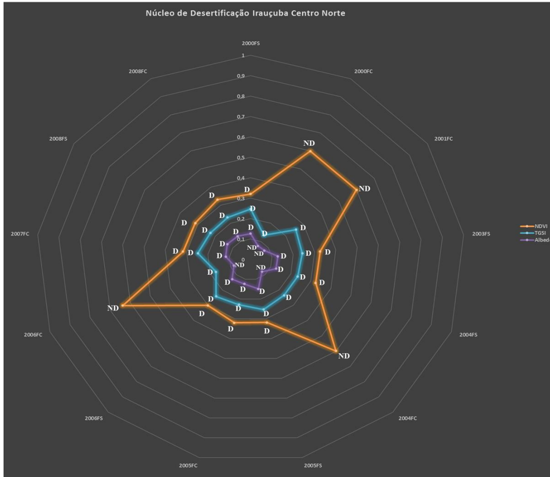
Figura 45 - NDVI, TGSi e Albedo para o núcleo entre os anos de 2000 a 2008
